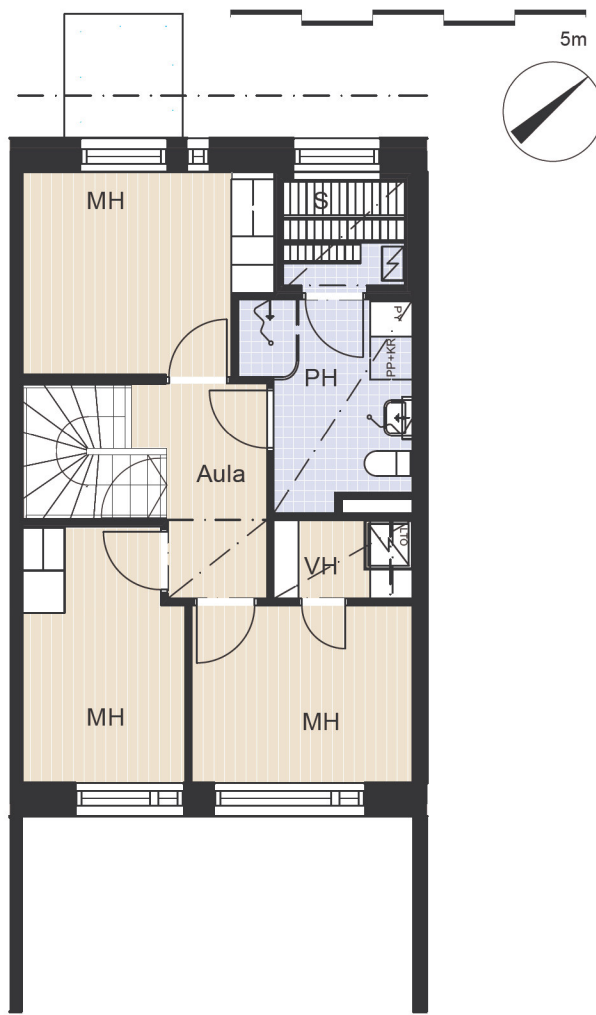
2. KERROS
