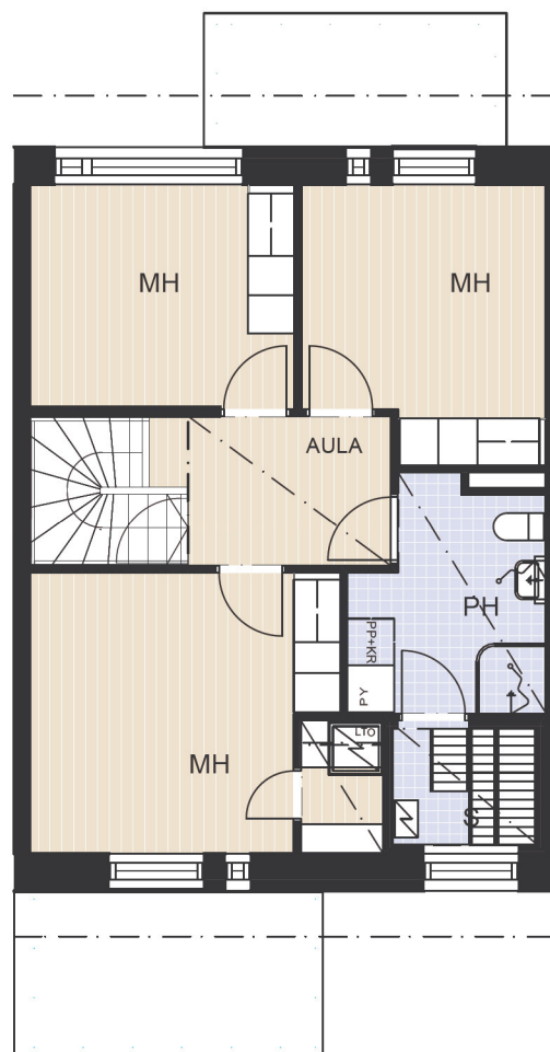
2. KERROS
