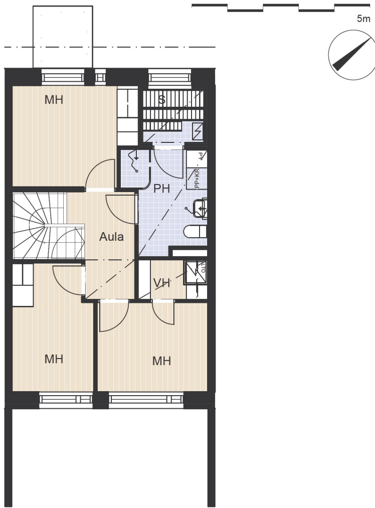
2. KERROS
