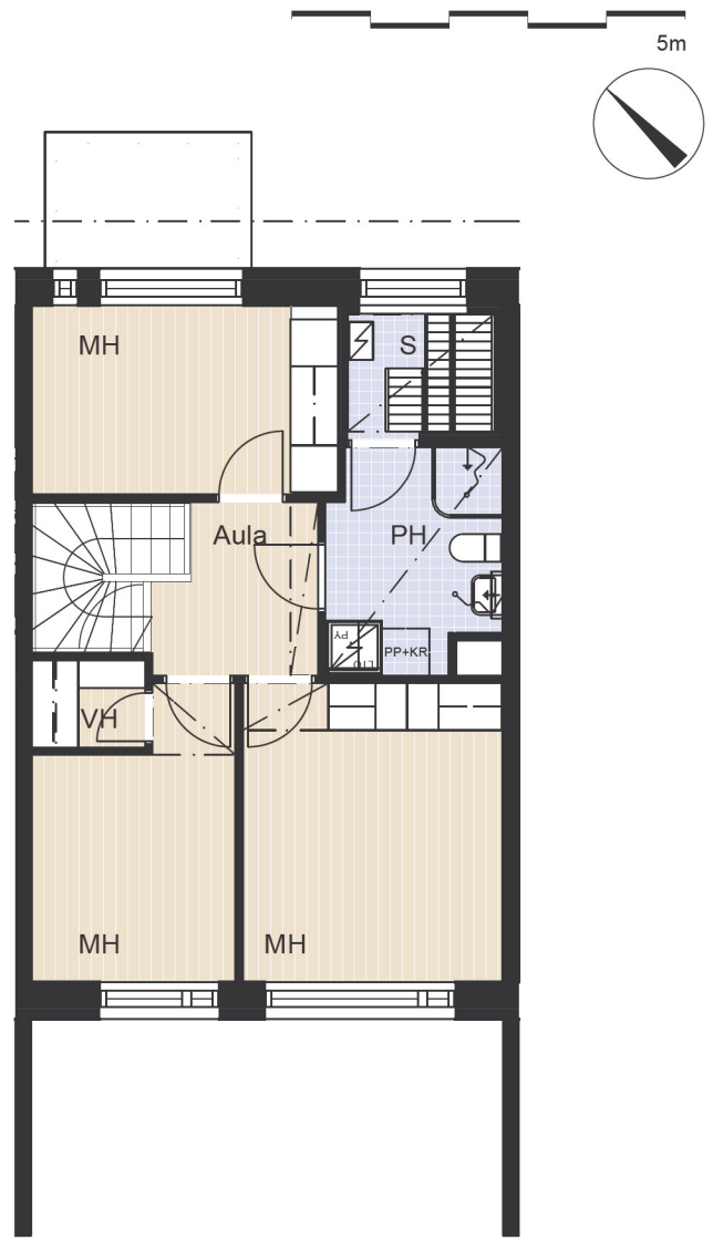
2. KERROS
