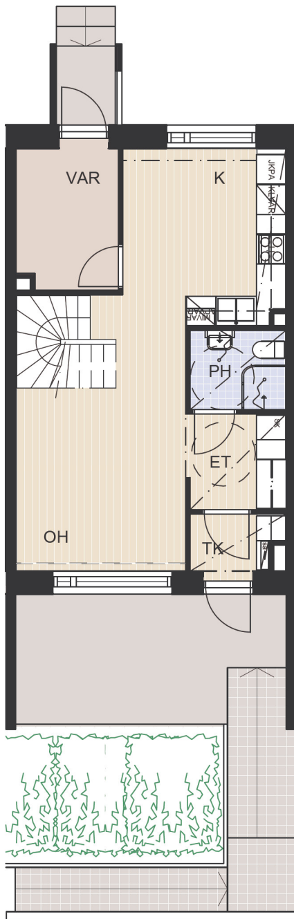
1. KERROS
