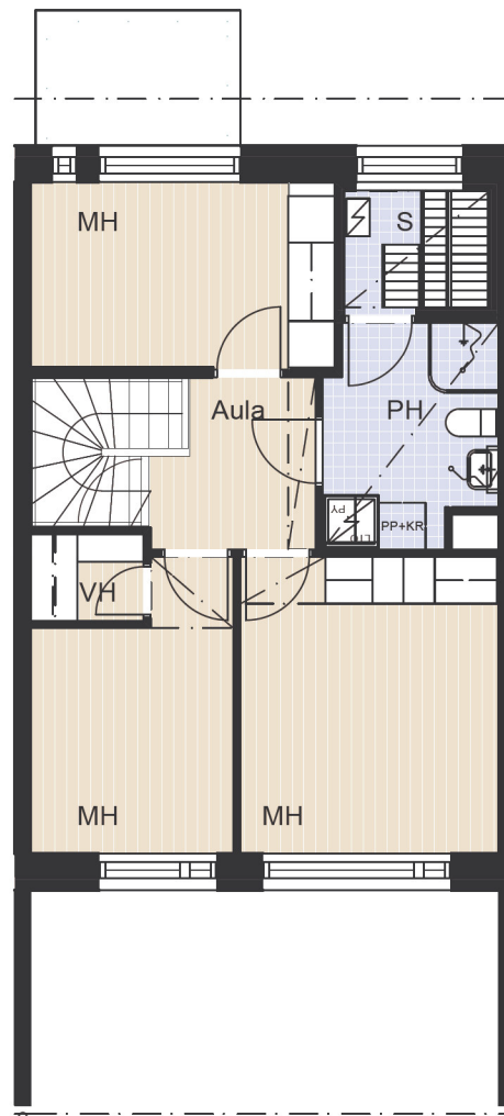
2. KERROS
