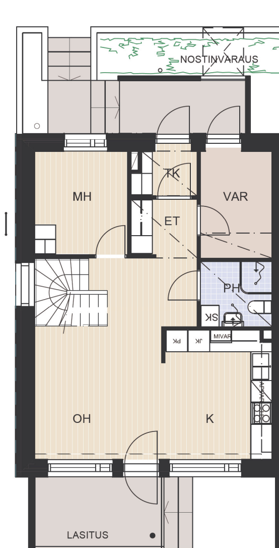
1. KERROS
