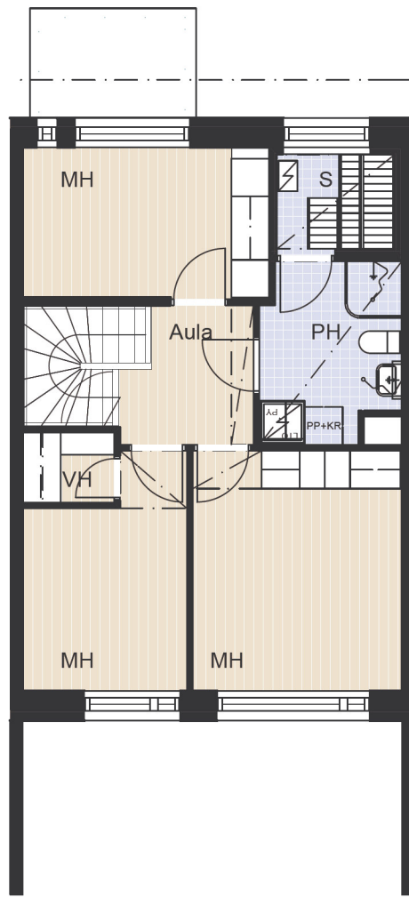
2. KERROS
