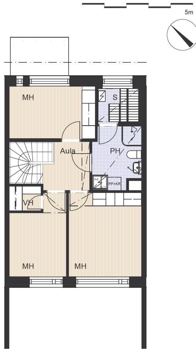
2. KERROS
