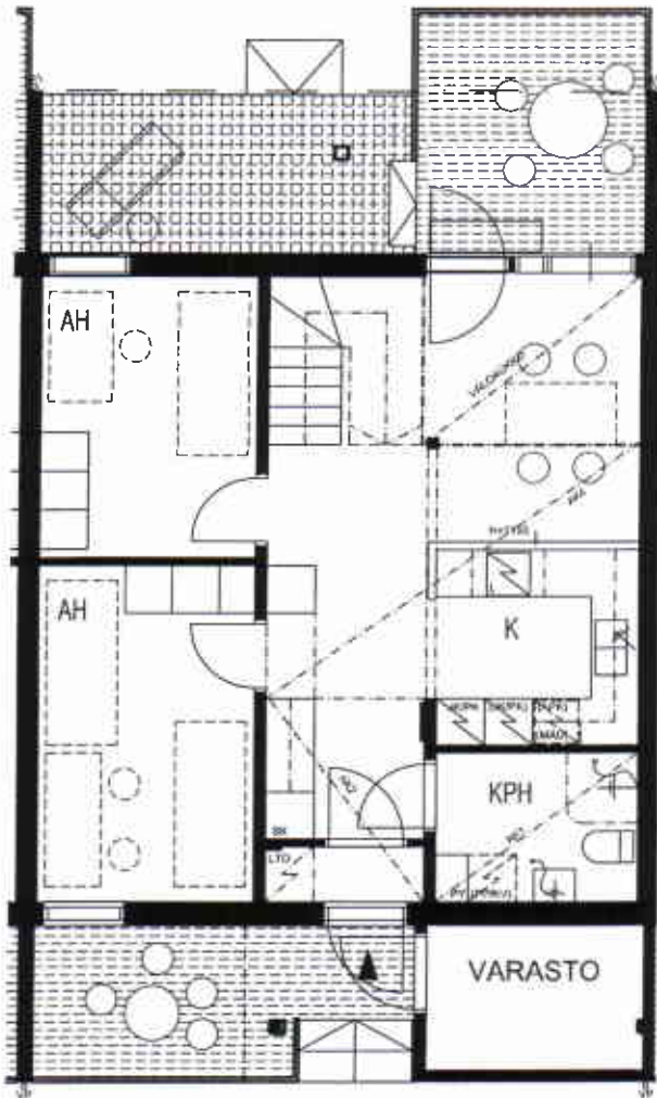
1. KERROS
