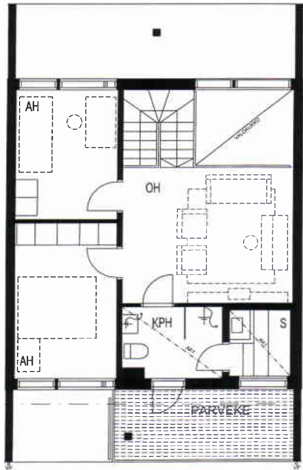
2. KERROS
