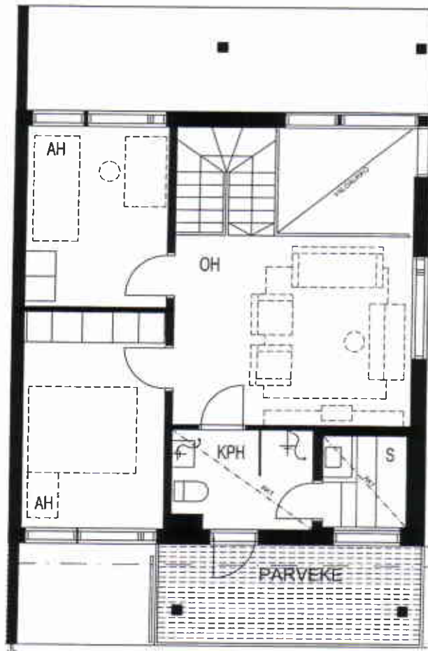
2. KERROS
