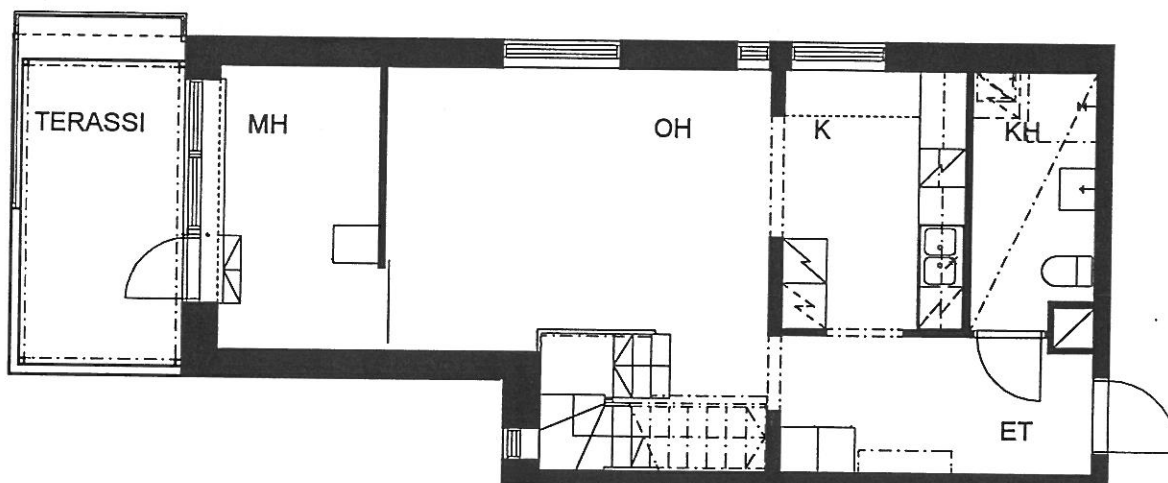
ALAKERTA 4. KERROS
