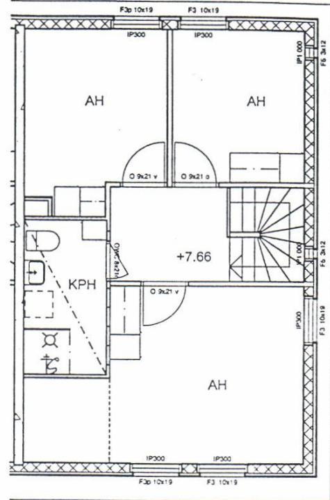
2.KERROS
