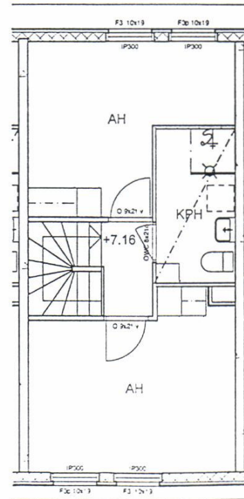
2.KERROS
