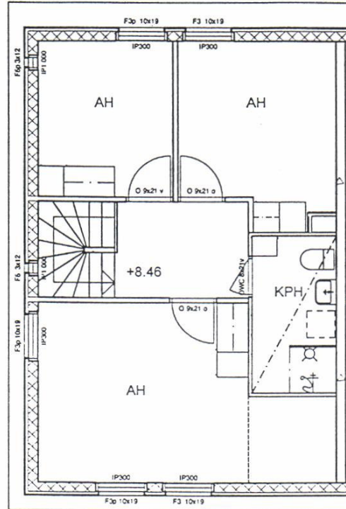
2.KERROS
