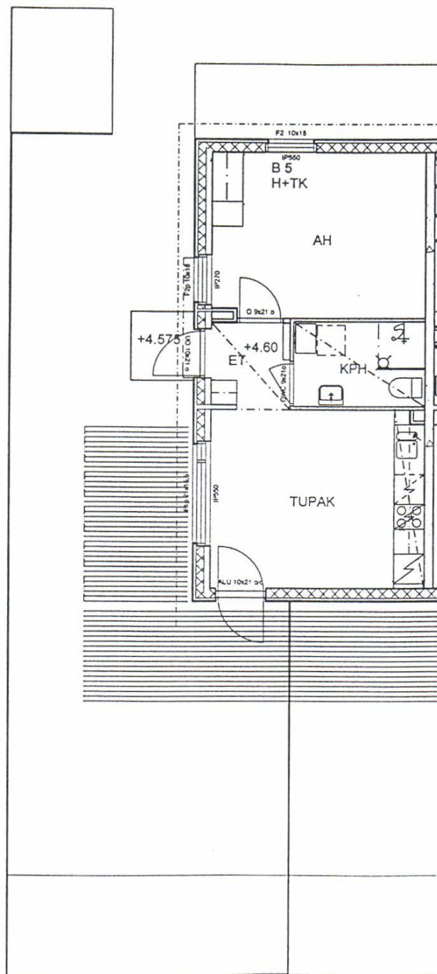
1.KERROS
