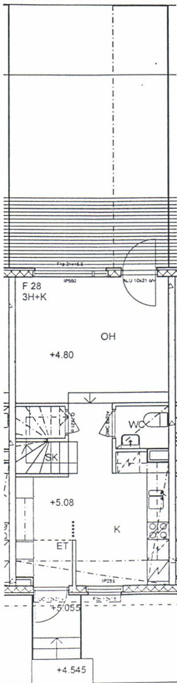
1.KERROS
