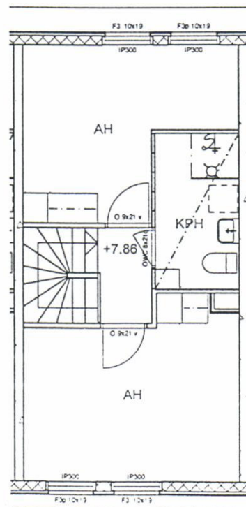
2.KERROS
