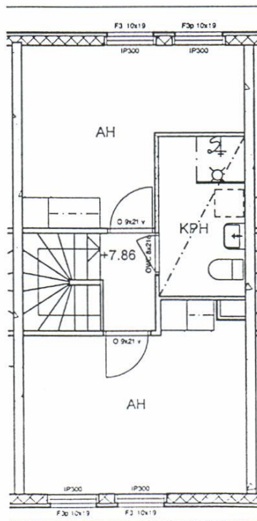
2.KERROS
