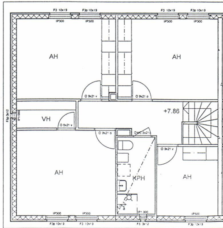
2.KERROS
