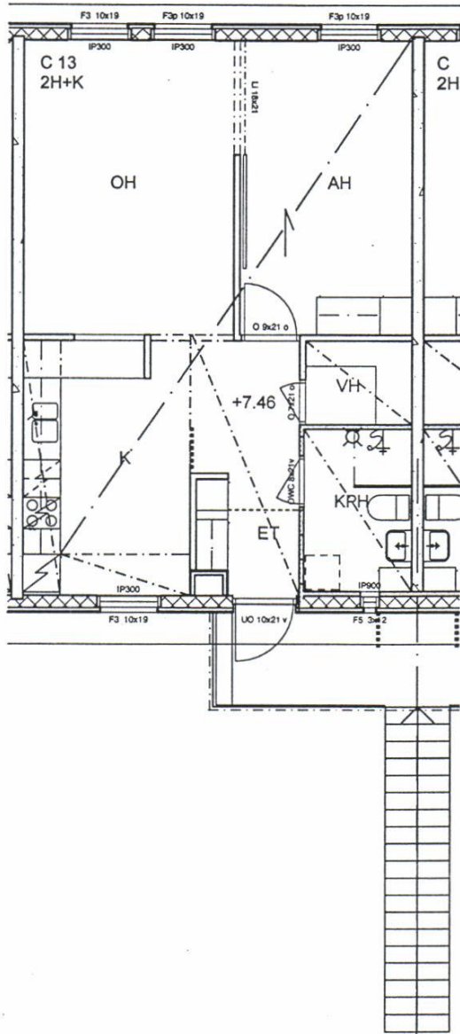
2.KERROS
