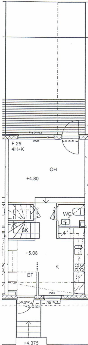
1.KERROS
