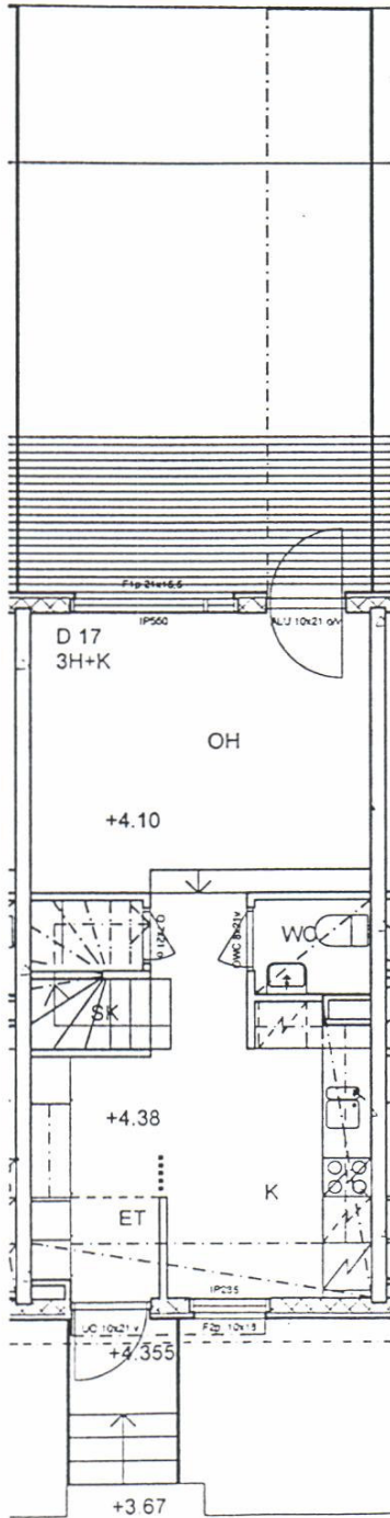
1.KERROS
