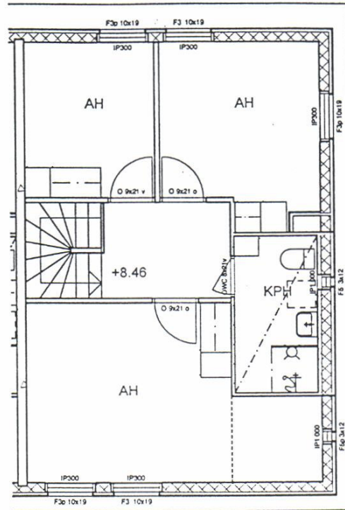
2.KERROS
