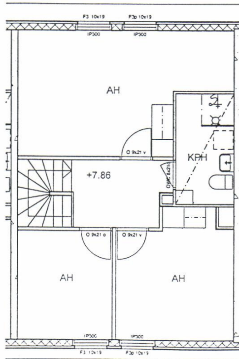
2.KERROS
