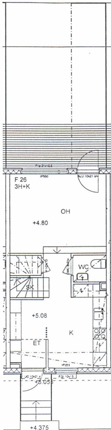
1.KERROS
