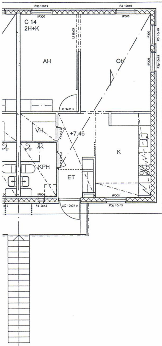
2.KERROS
