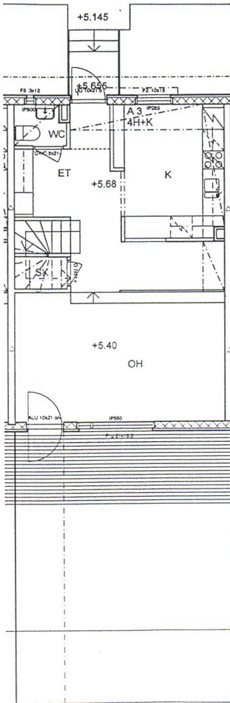
1.KERROS
