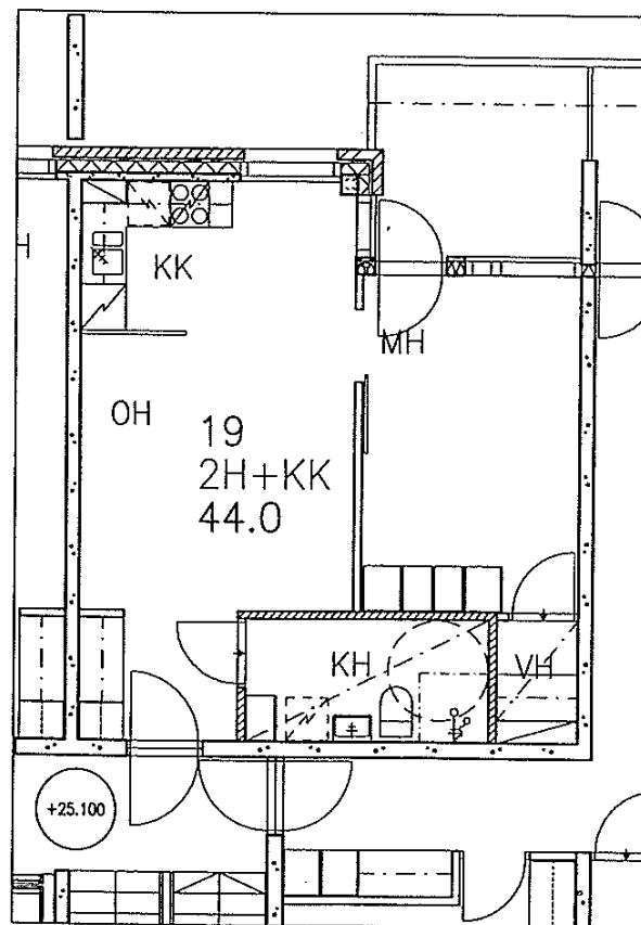
2H+KK 5. KERROS 1:100 04.06.1998
