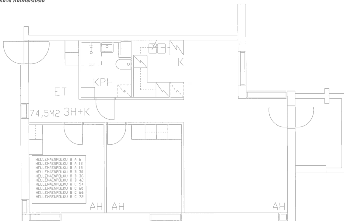
Pohjakuva huoneistosta
