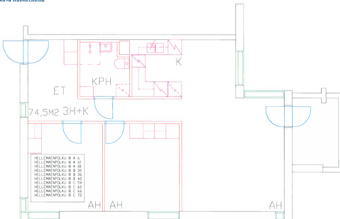
Pohjakuva huoneistosta
