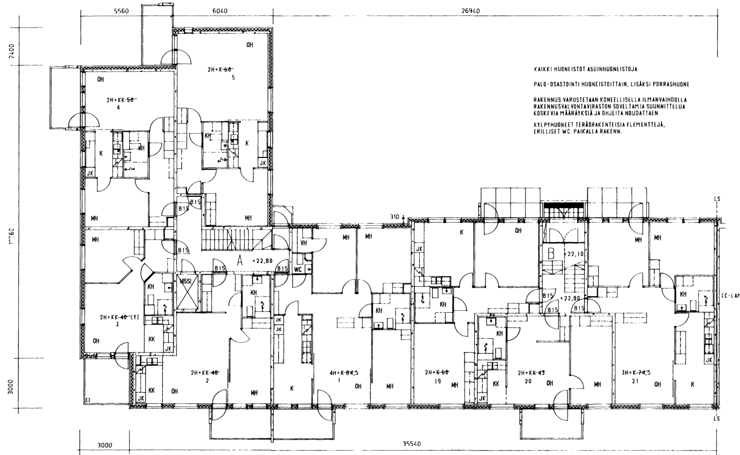
RAKENNUSPIIRUSTUKSESSA No 5
