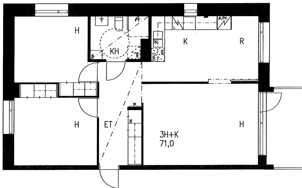
2. KERROS
