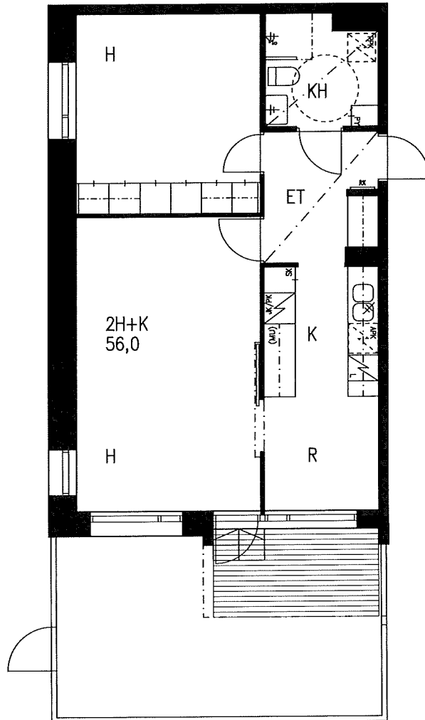
1. KERROS
