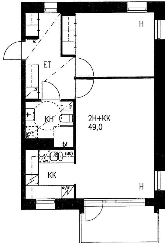
3. KERROS
