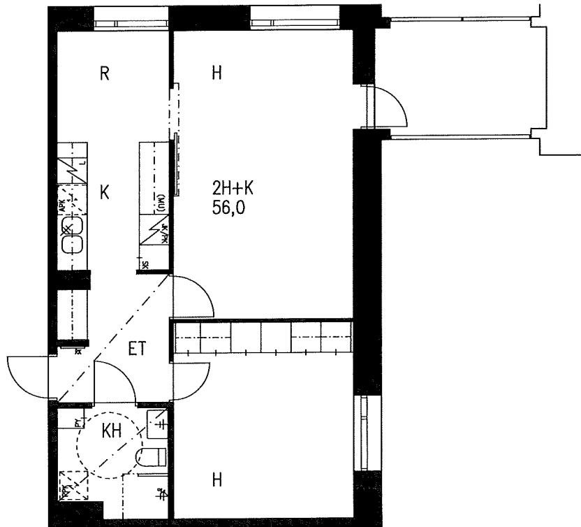
2. KERROS
