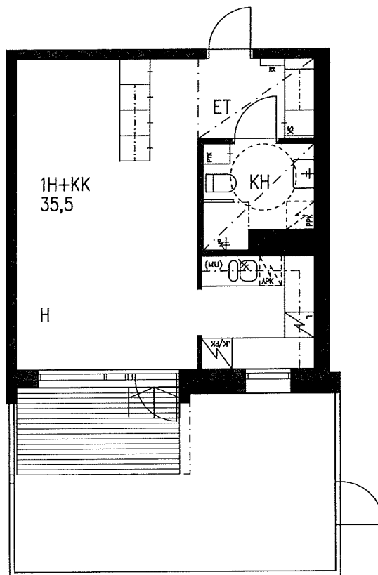
1. KERROS
