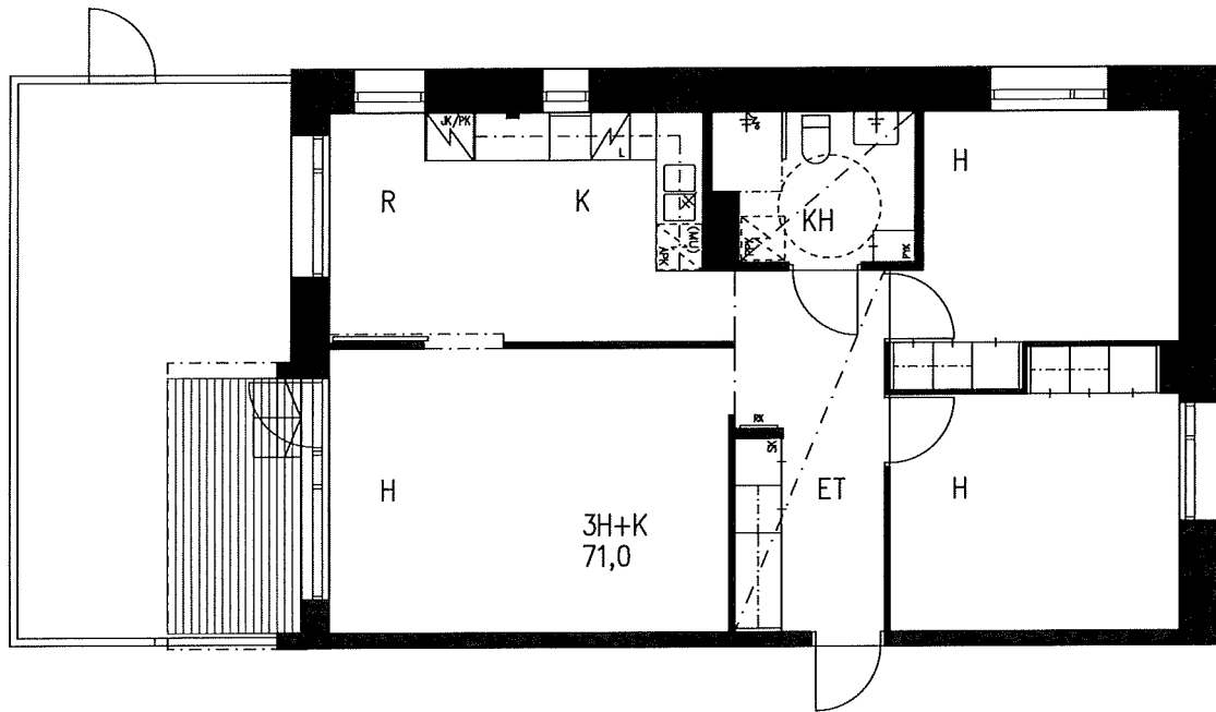
1. KERROS
