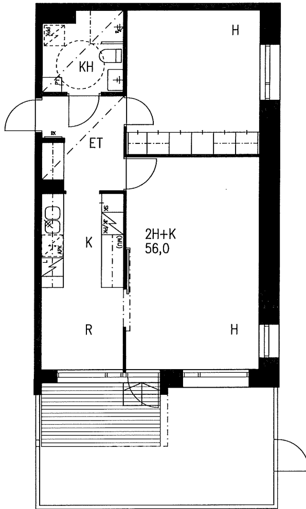
1. KERROS
