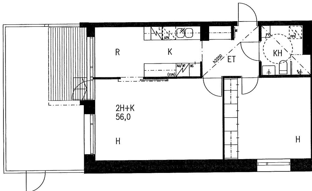
1. KERROS
