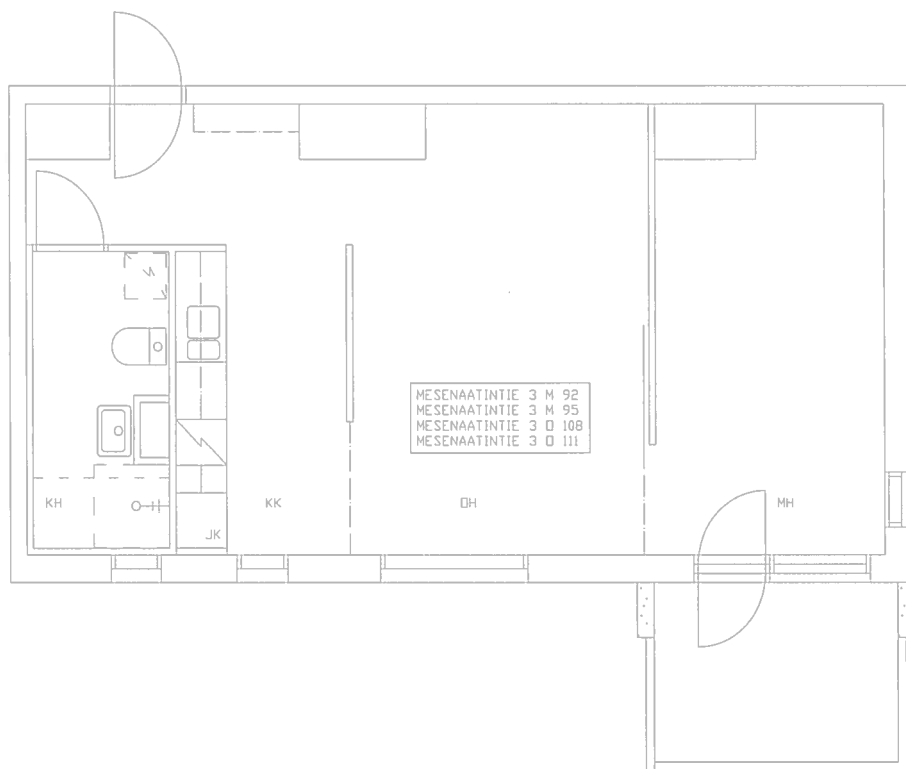
Pohjakuva huoneistosta
