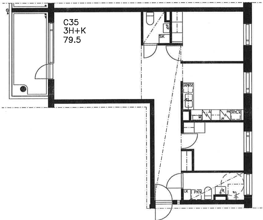
POHJAPIIRUSTUS 1/100
