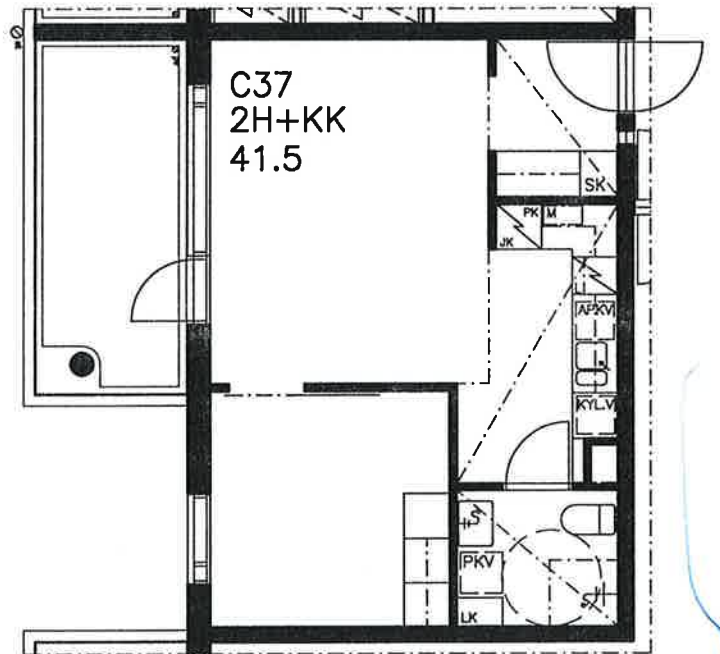
POHJAPIIRUSTUS 1/100
