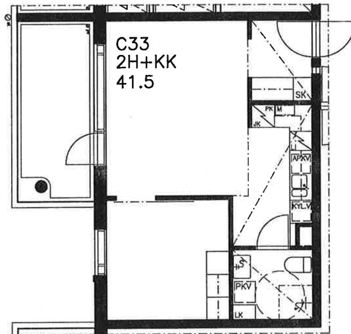
POHJAPIIRUSTUS 1/100
