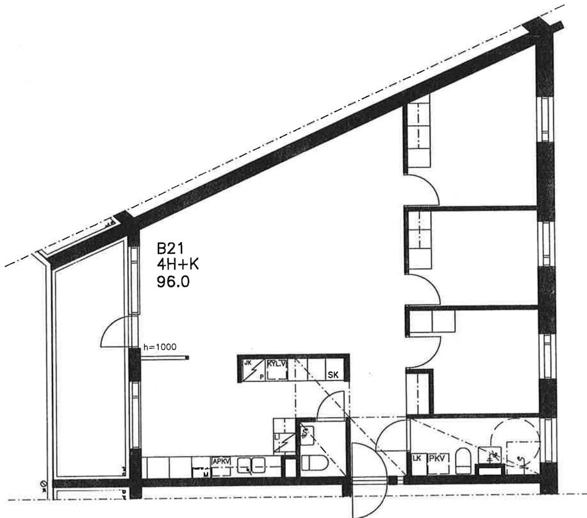
POHJAPIIRUSTUS 1/100
