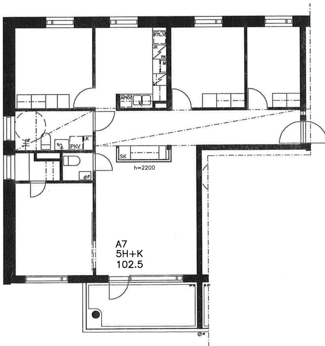
POHJAPIIRUSTUS 1/100
