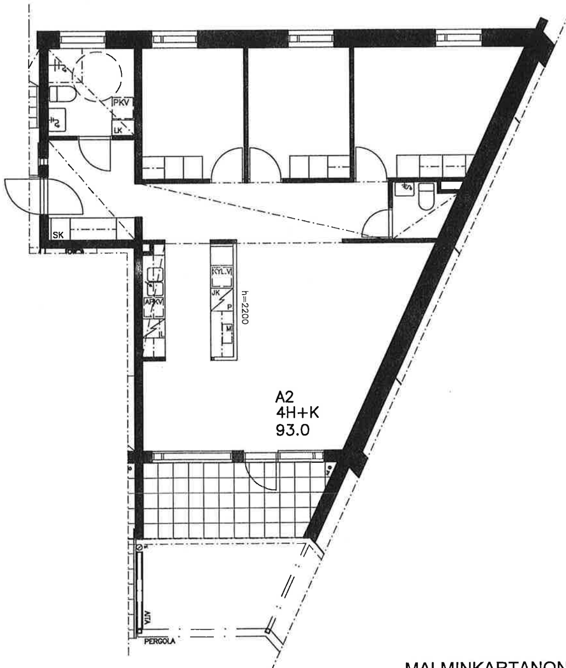
POHJAPIIRUSTUS 1/100
