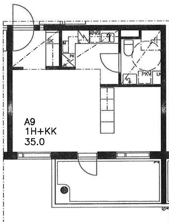
POHJAPIIRUSTUS 1/100
