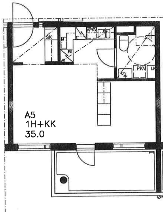
POHJAPIIRUSTUS 1/100
