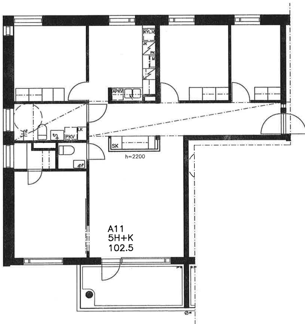
POHJAPIIRUSTUS 1/100
