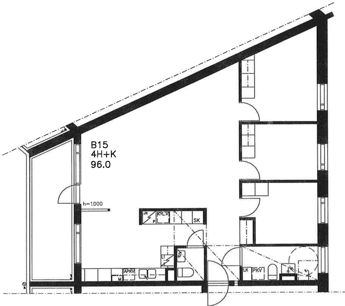
POHJAPIIRUSTUS 1/100
