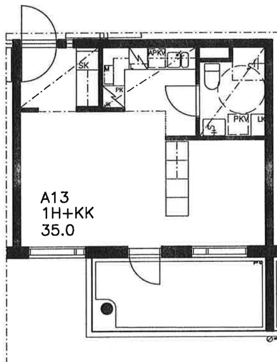
POHJAPIIRUSTUS 1/100
