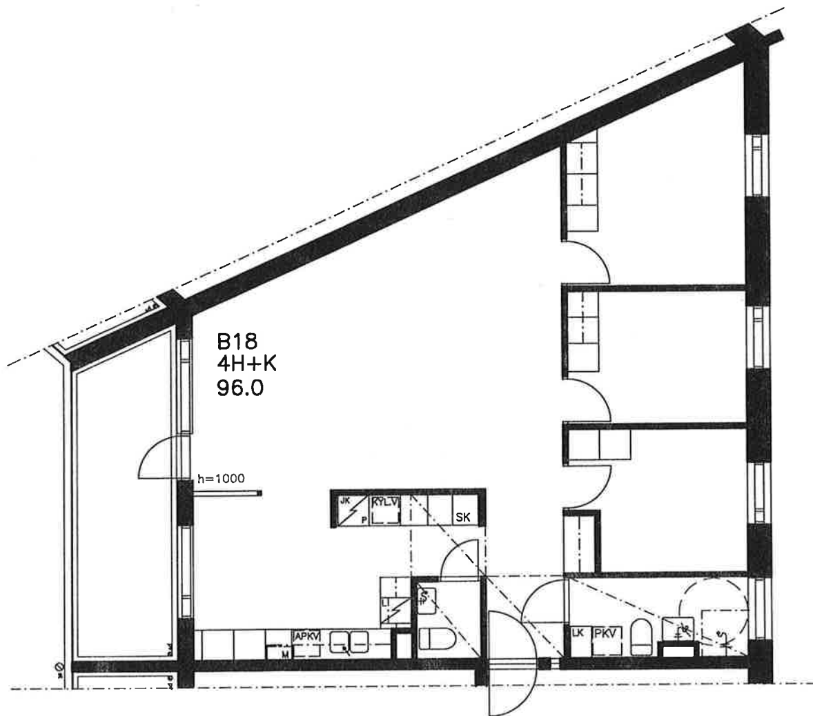
POHJAPIIRUSTUS 1/100
