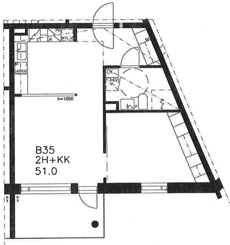
POHJAPIIRUSTUS 1/100
