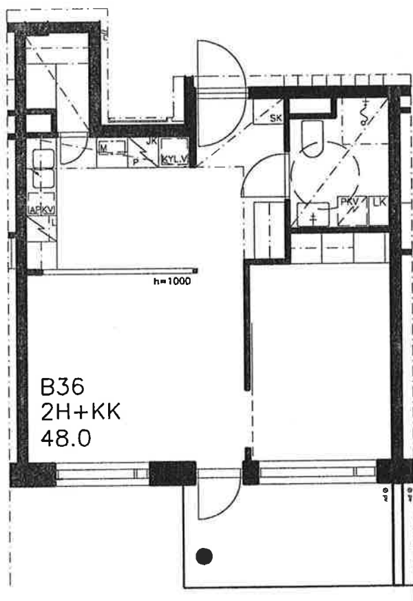
POHJAPIIRUSTUS 1/100
