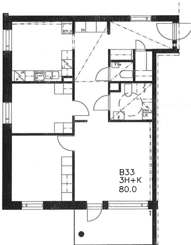
POHJAPIIRUSTUS 1/100
