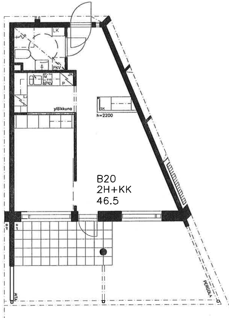
POHJAPIIRUSTUS 1/100
