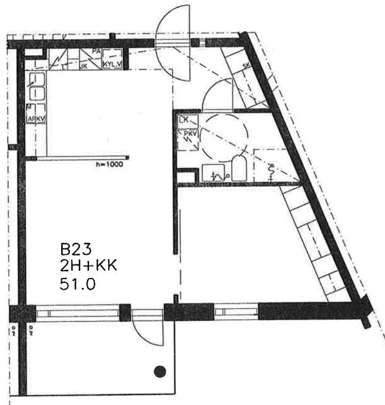
POHJAPIIRUSTUS 1/100
