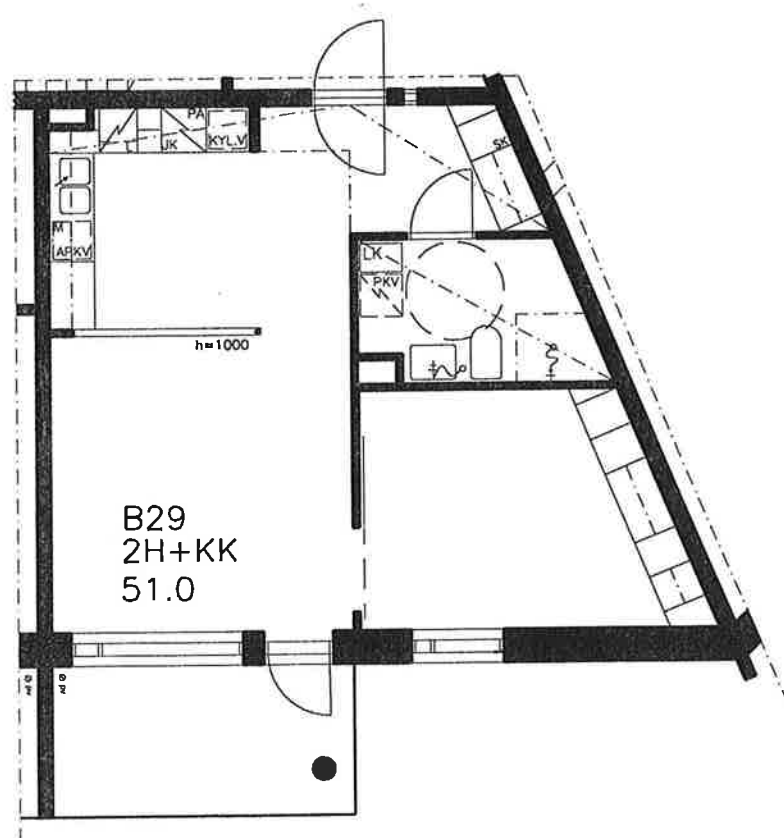
POHJAPIIRUSTUS 1/100
