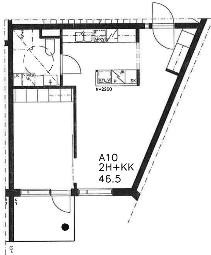
POHJAPIIRUSTUS 1/100
