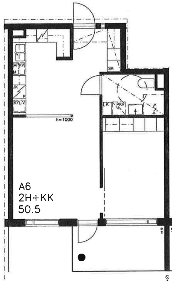
POHJAPIIRUSTUS 1/100
