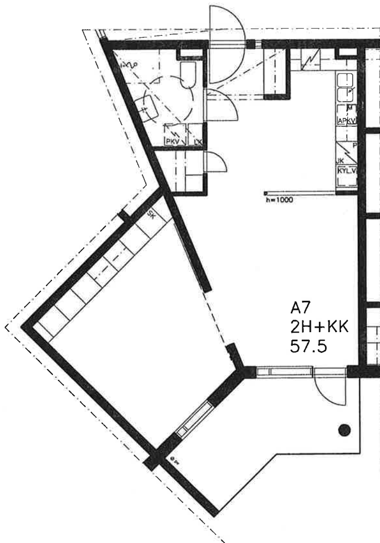
POHJAPIIRUSTUS 1/100
