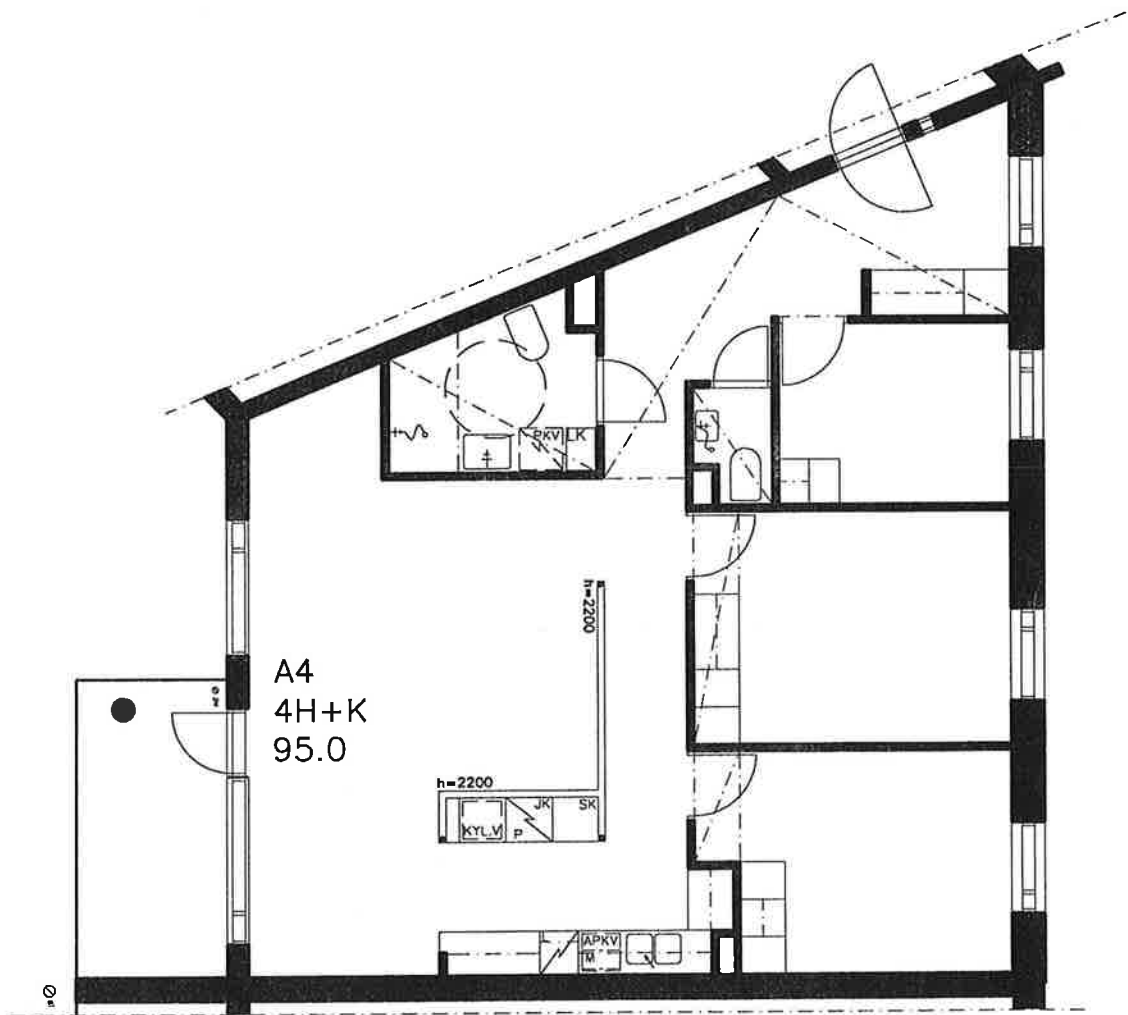
POHJAPIIRUSTUS 1/100
