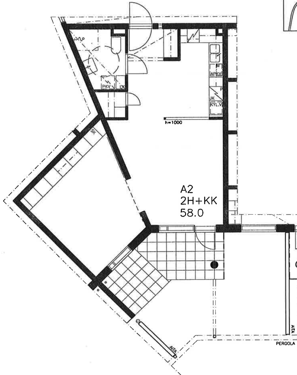
POHJAPIIRUSTUS 1/100
