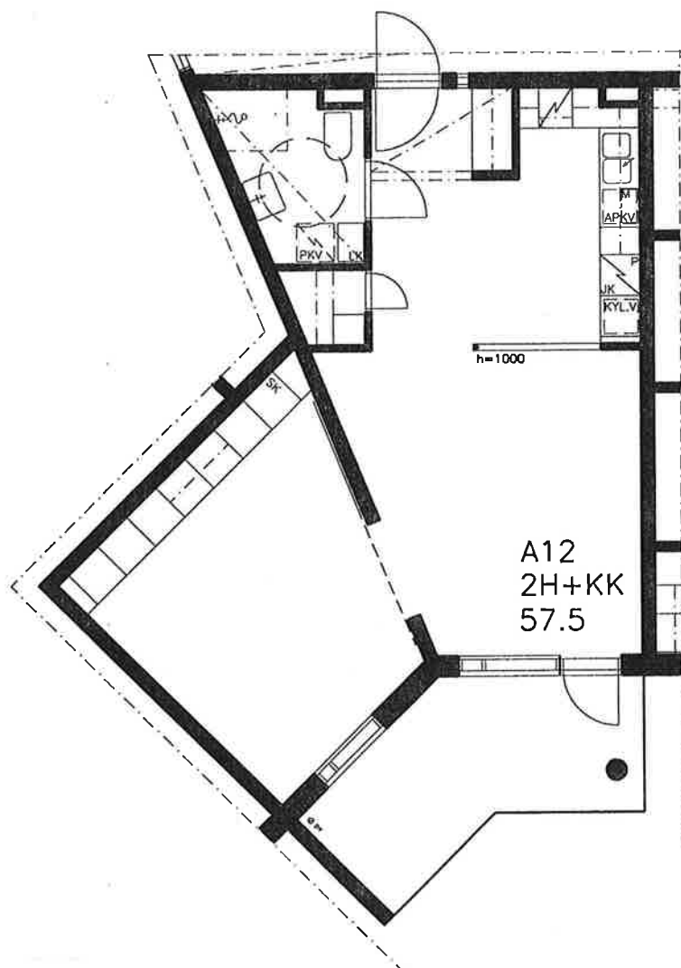
POHJAPIIRUSTUS 1/100
