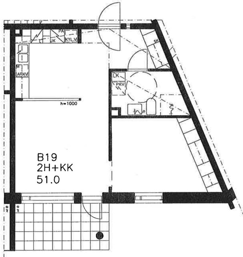
POHJAPIIRUSTUS 1/100
