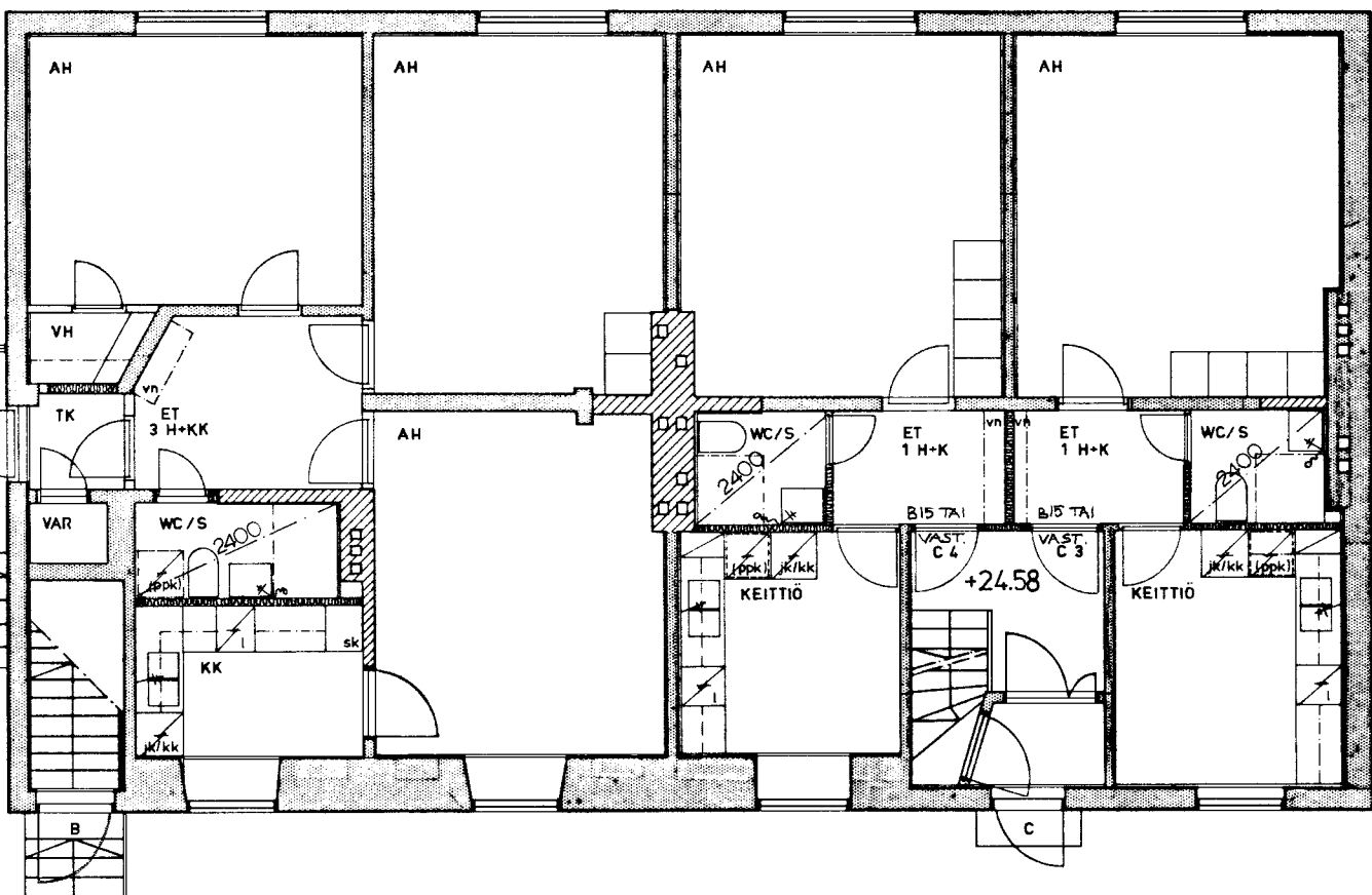
1. KERROS
