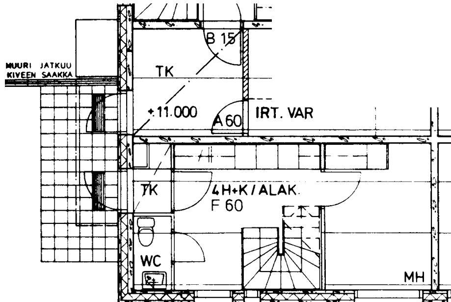
1. KERROS
