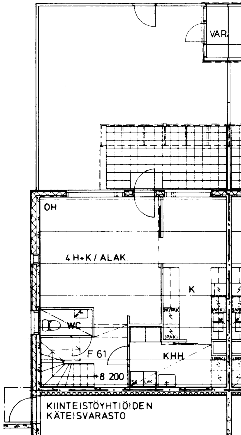
POHJAKERROS
