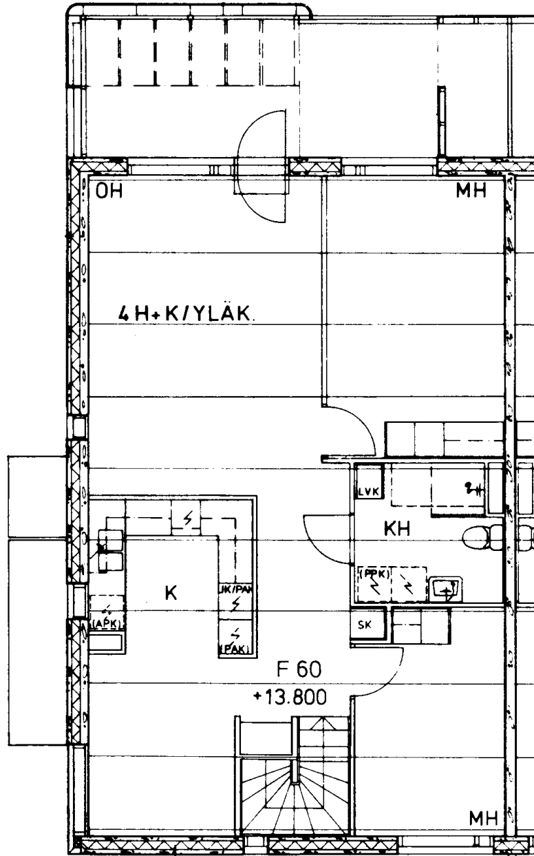
2. KERROS
