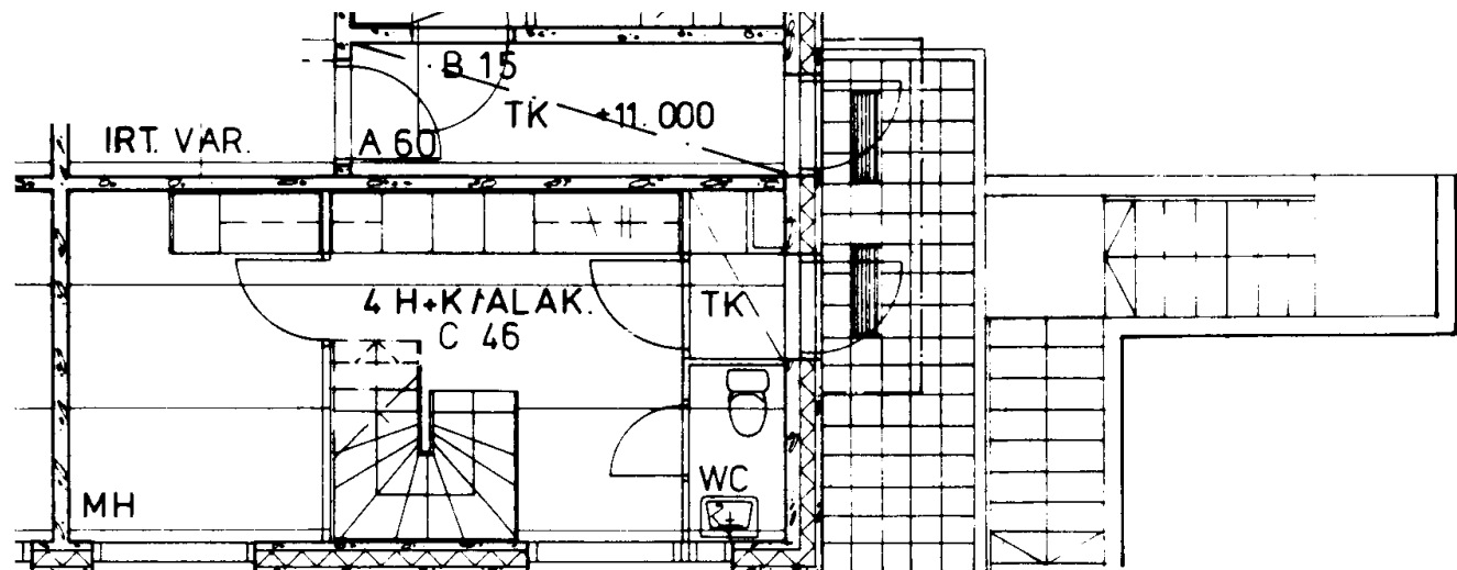
1. KERROS
