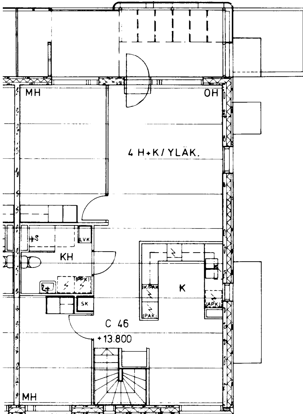
2. KERROS
