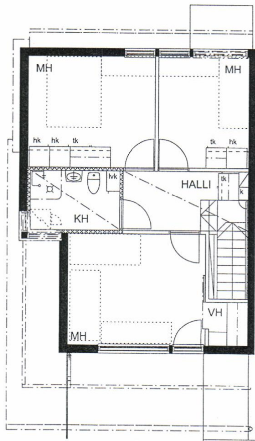
POHJA 2. krs 1:100
