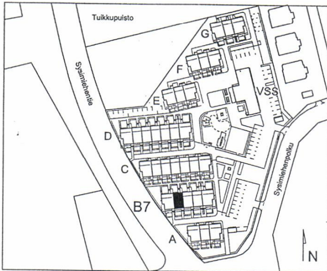
ASEMAPIIRROS 1:2000
