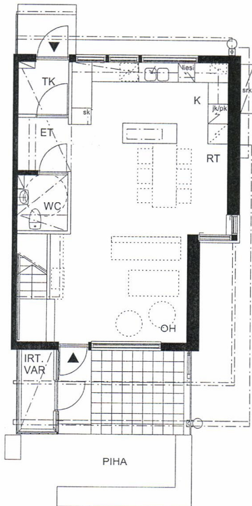
POHJA 1. krs 1:100
