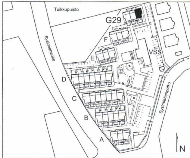
ASEMAPIIRROS 1 :2000
