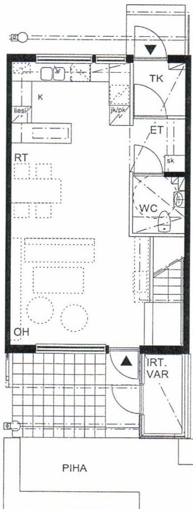
POHJA 1. krs 1:100
