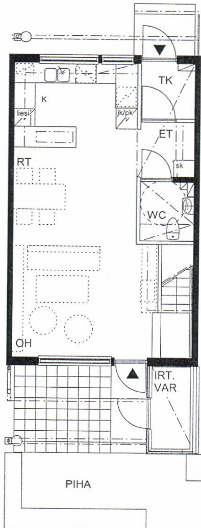
POHJA 1. krs 1:100
