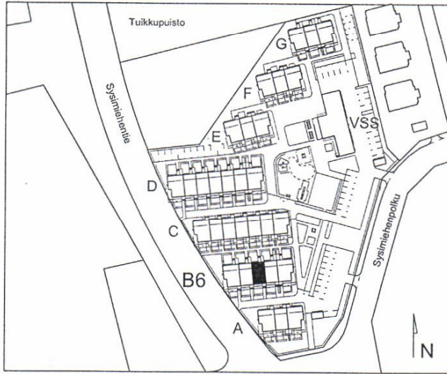
ASEMAPIIRROS 1 :2000
