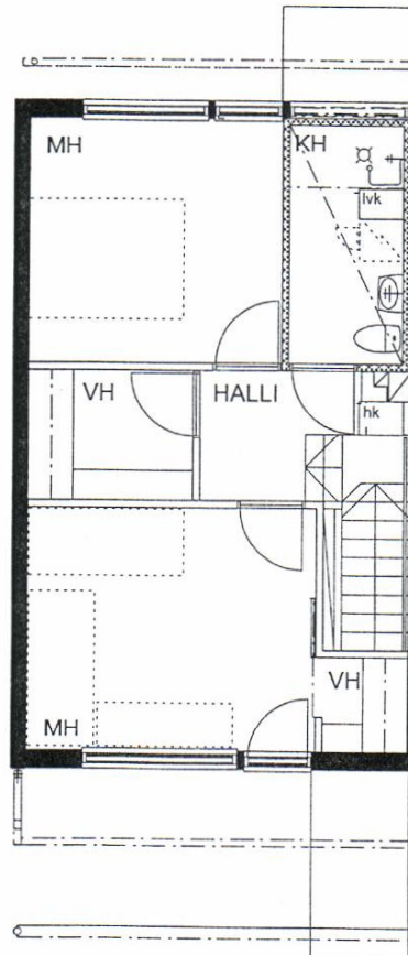
POHJA 2. krs 1:100
