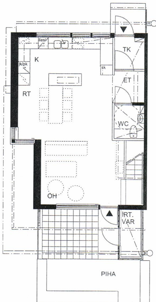
POHJA 1. krs 1:100
