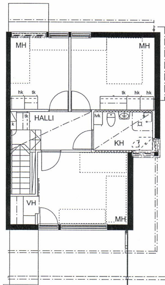
POHJA 2. krs 1:100
