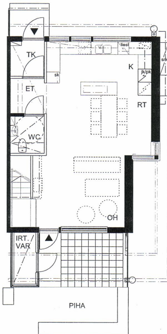
POHJA 1. krs 1:100
