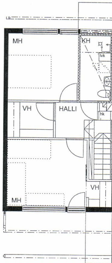
POHJA 2. krs 1:100
