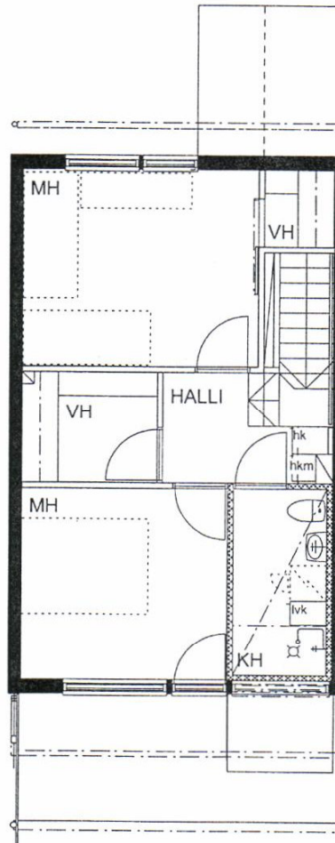
POHJA 2. krs 1:100
