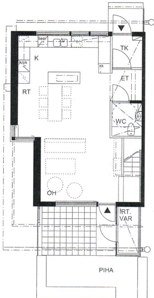
POHJA 1. krs 1:100
