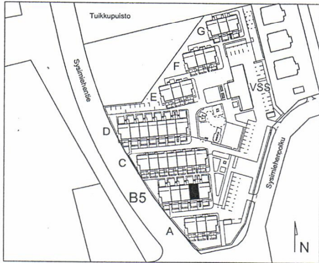
ASEMAPIIRROS 1:2000
