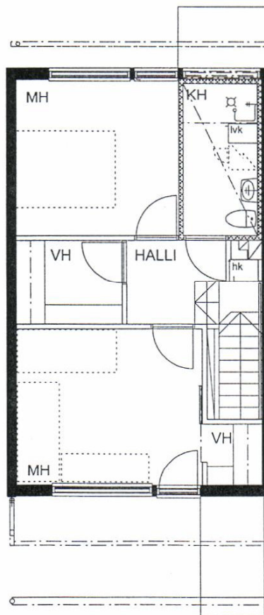
POHJA 2. krs 1:100
