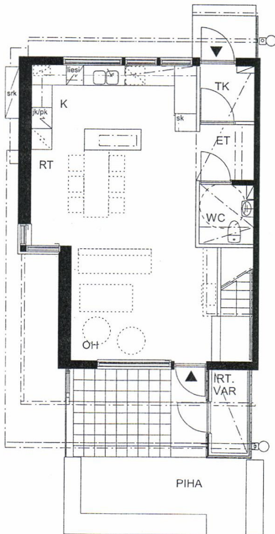
POHJA 1. krs 1:100
