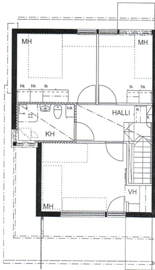
POHJA 2. krs 1:100
