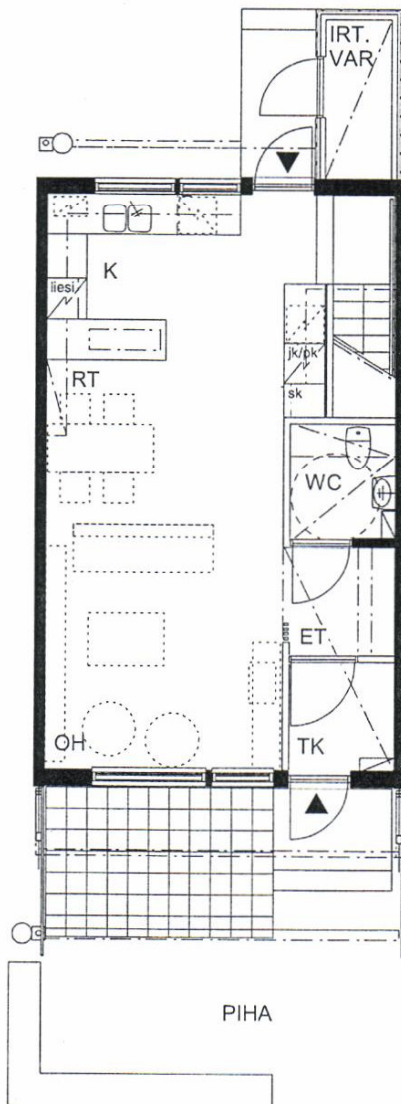
POHJA 1. krs 1:100
