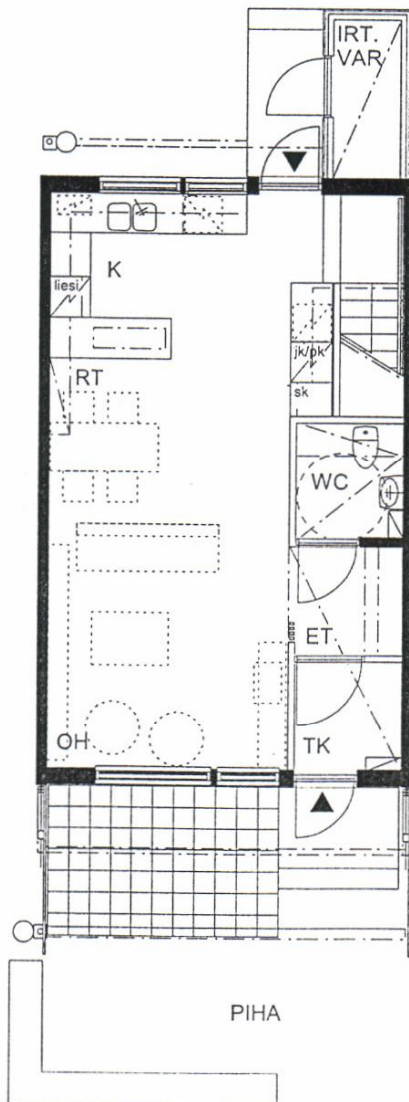
POHJA 1. krs 1:100
