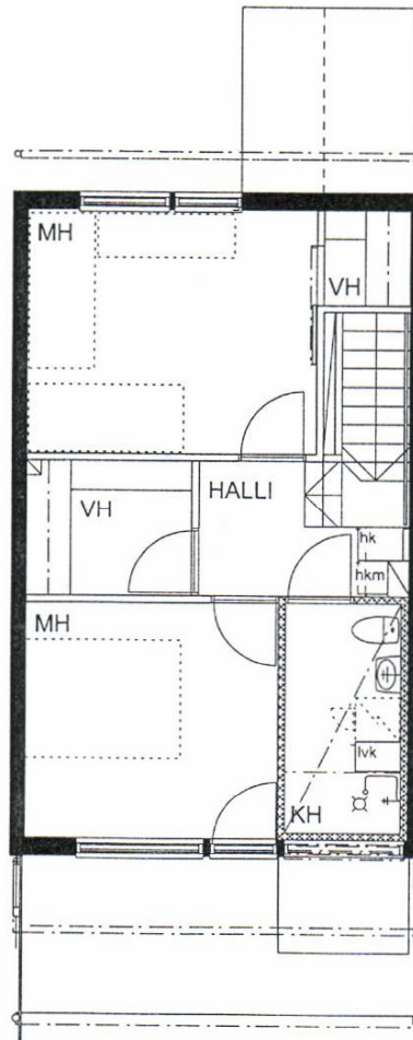
POHJA 2. krs 1:100
