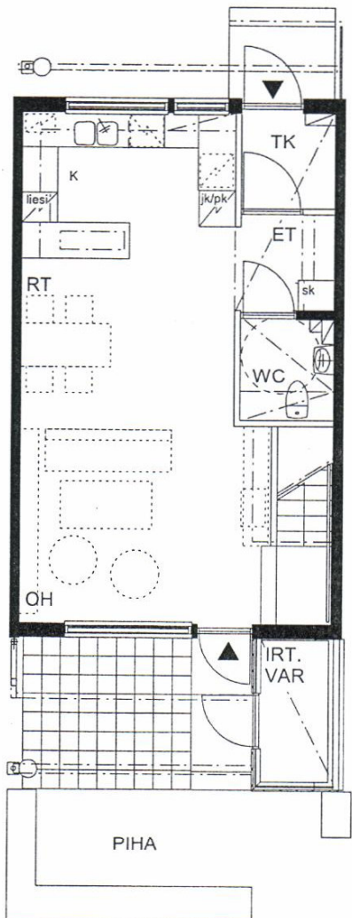
POHJA 1. krs 1:100
