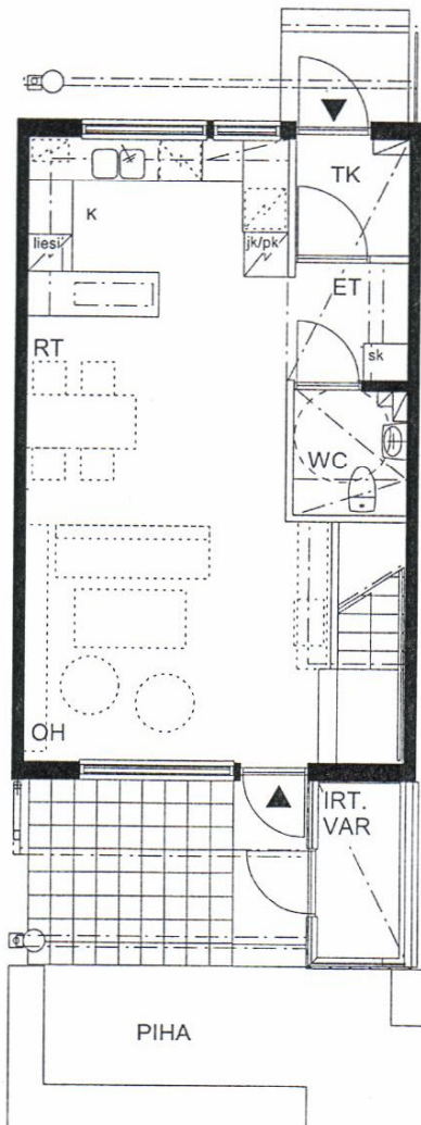
POHJA 1. krs 1:100
