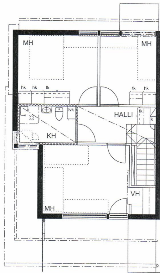
POHJA 2. krs 1:100
