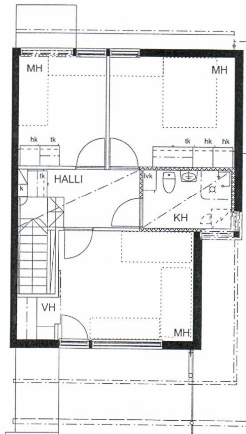
POHJA 2. krs 1:100
