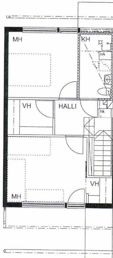
POHJA 2. krs 1:100
