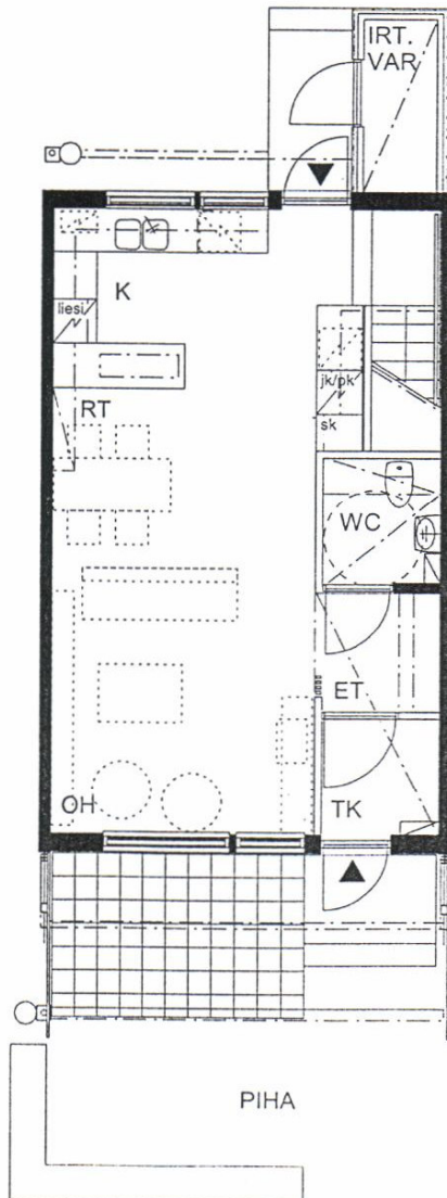
POHJA 1. krs 1:100
