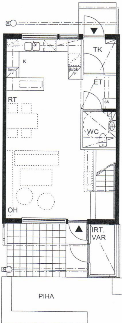
POHJA 1. krs 1:100
