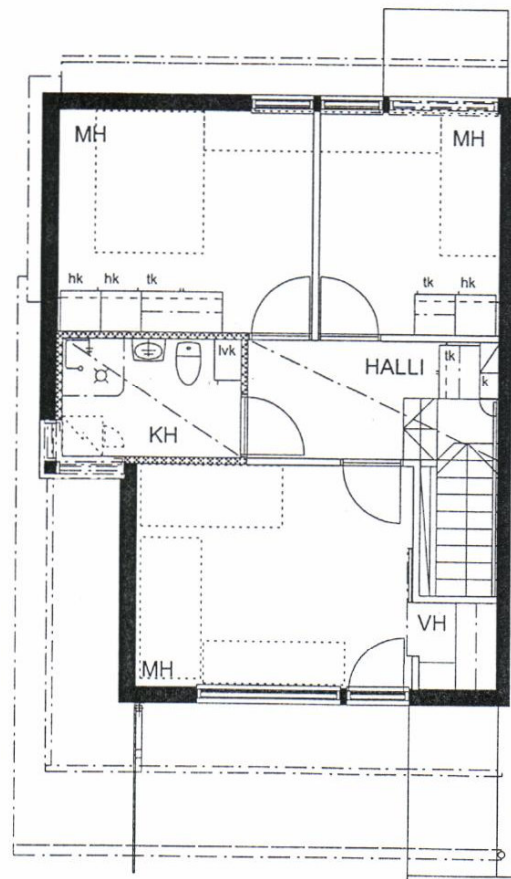
POHJA 2. krs 1:100
