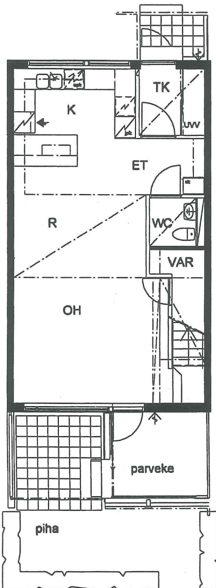
POHJA 1. krs 1:100
