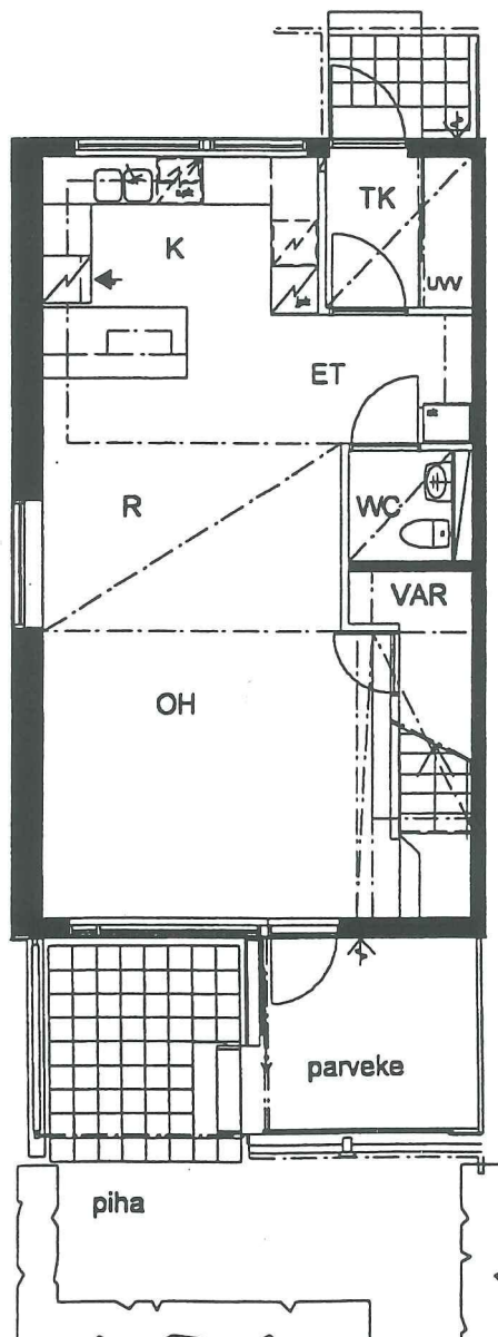
POHJA 1. krs 1:100
