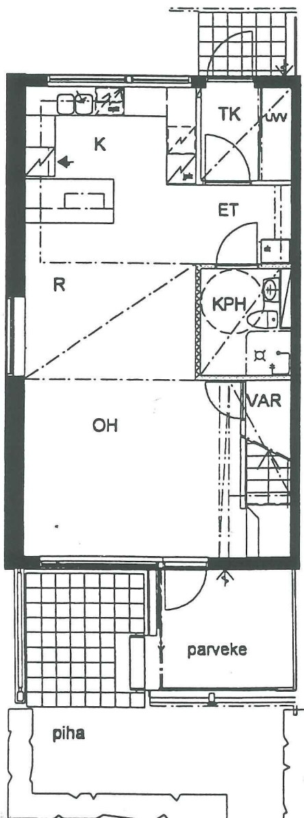
POHJA 1. krs 1:100
