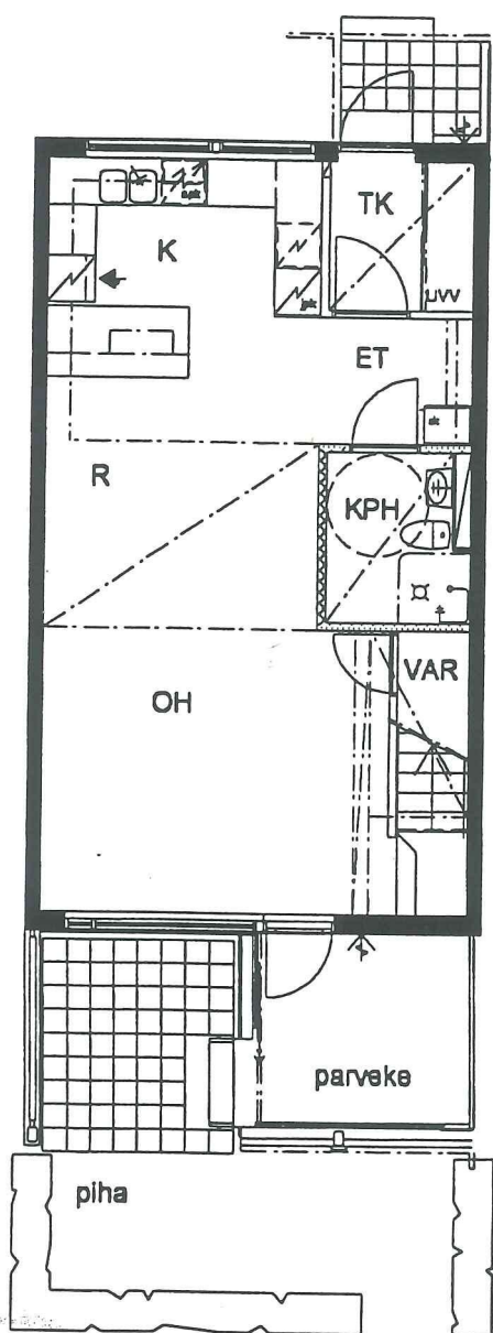
POHJA 1. krs 1:100
