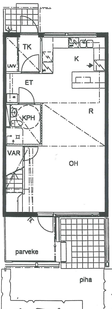
POHJA 1.krs 1:100
