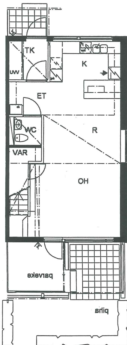
POHJA 1. krs 1:100
