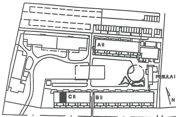
ASEMAPIIRROS 1:2000
