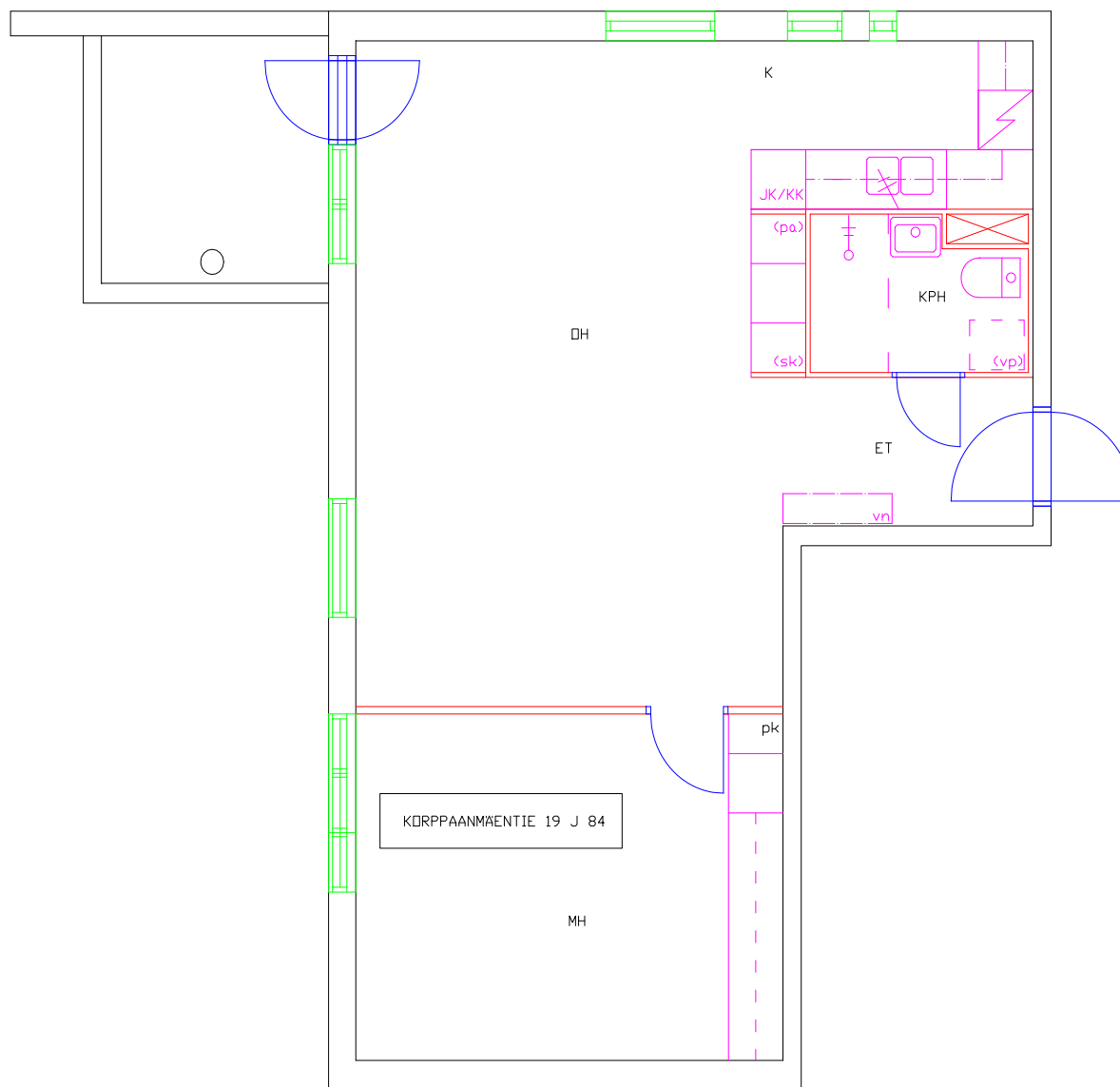
Pohjakuva huoneistosta
