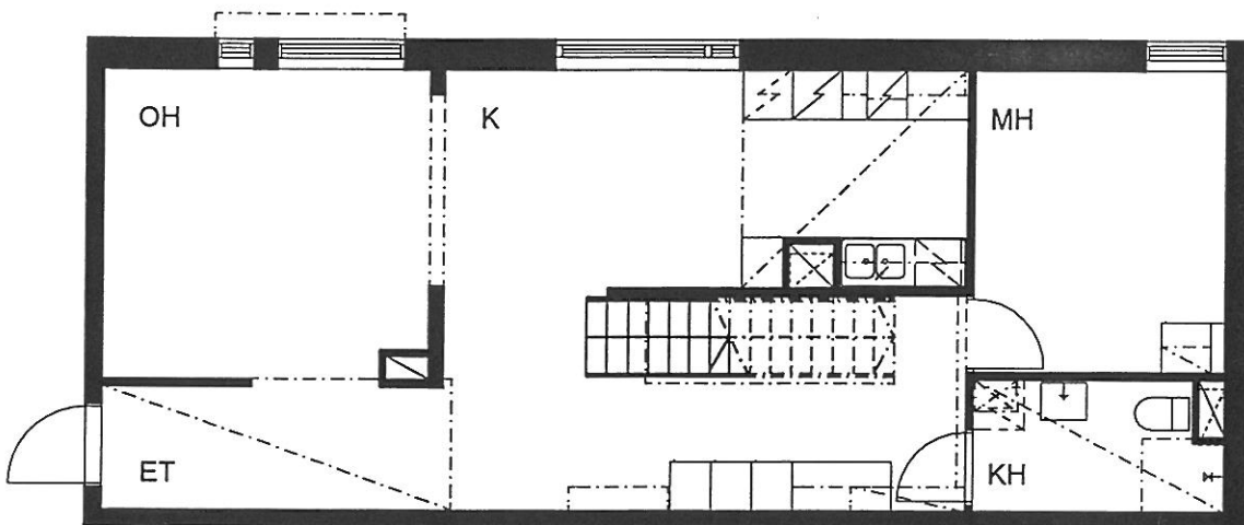
ALAKERTA 4. KERROS
