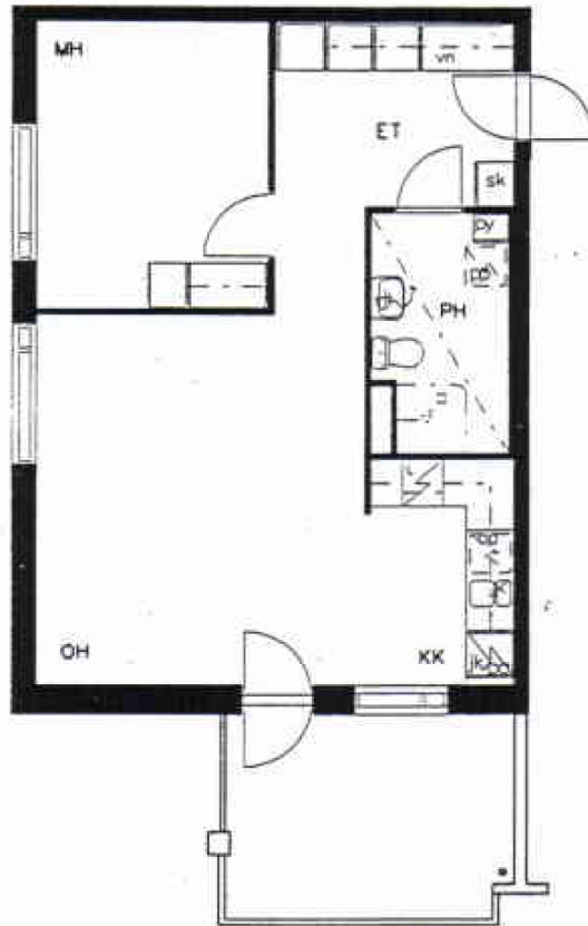
POHJAPIIRROS 1:100
