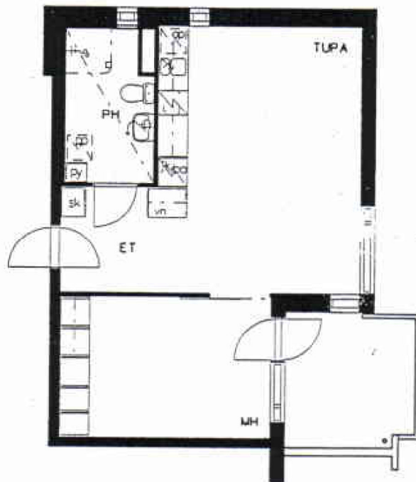
POHJAPIIRROS 1:100
