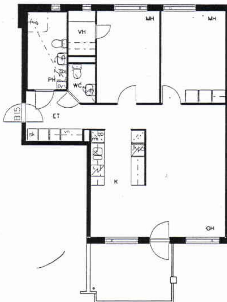
POHJAPIIRROS 1:100
