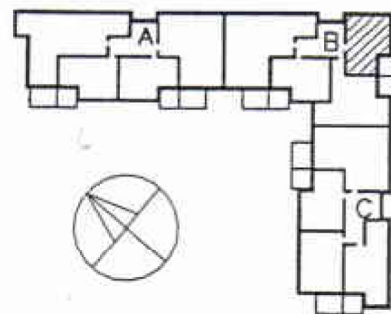
SIJANTIKAAVIO 2.- 6. KRS
