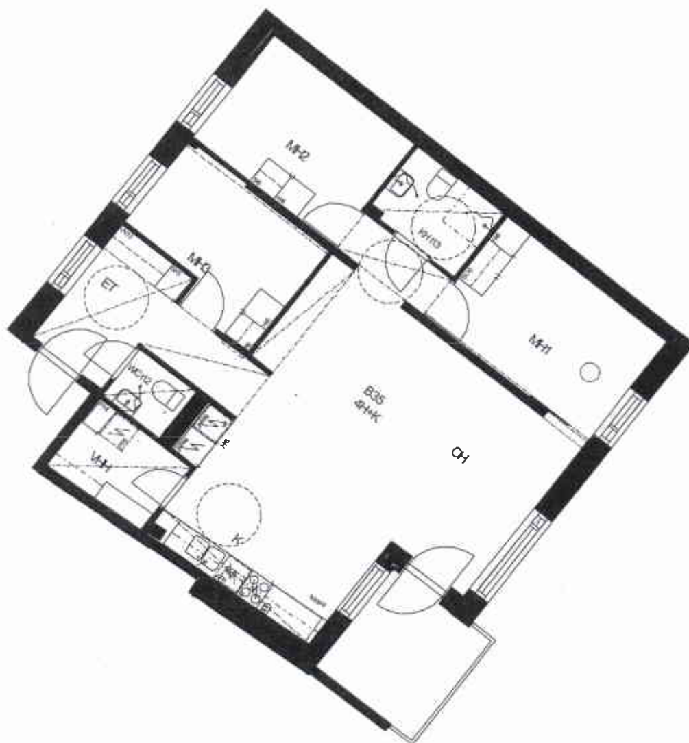
2.taso
