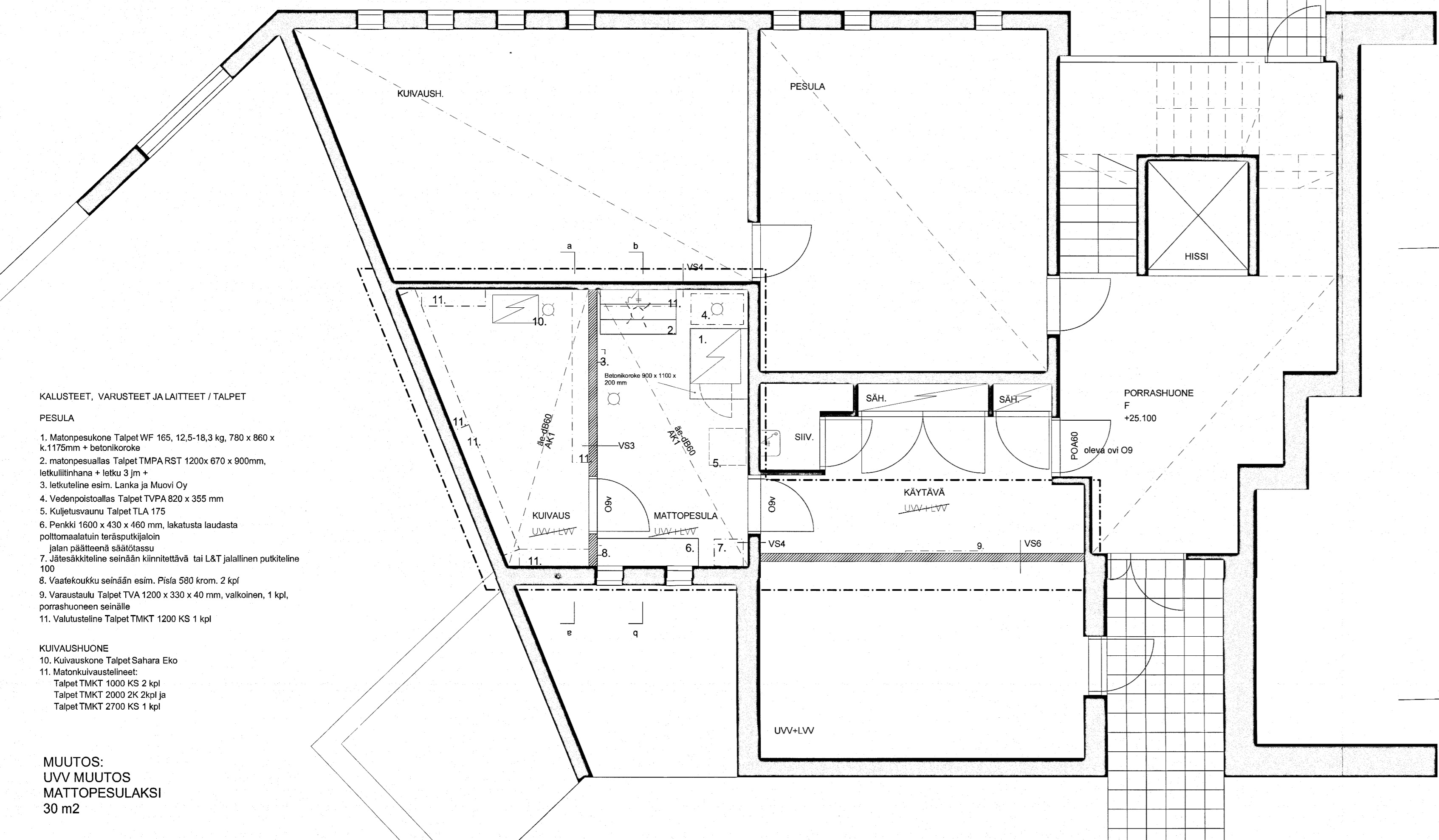
POHJA 1/50
