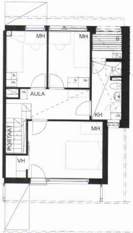
POHJA 2. KRS 1:100
