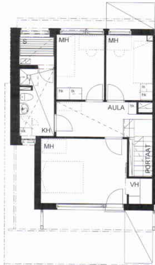
POHJA 2. KRS 1:100
