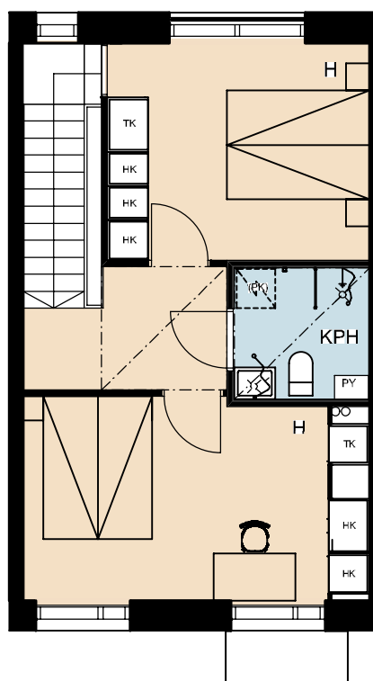
Huoneiston 2. krs
