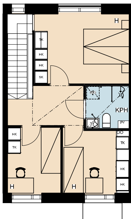
Huoneiston 2. krs
