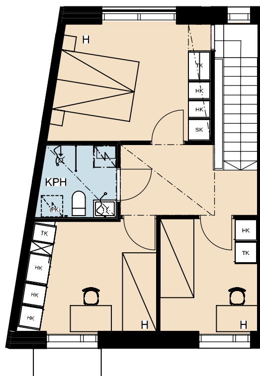
Huoneiston 2. krs
