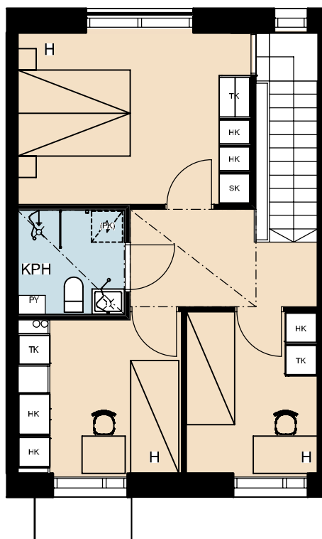
Huoneiston 2. krs
