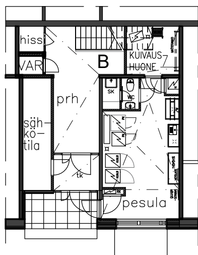
Kellarikerros
