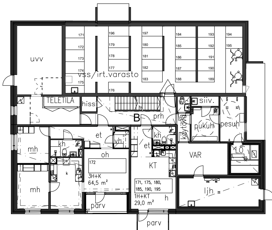
Maantasokerros
