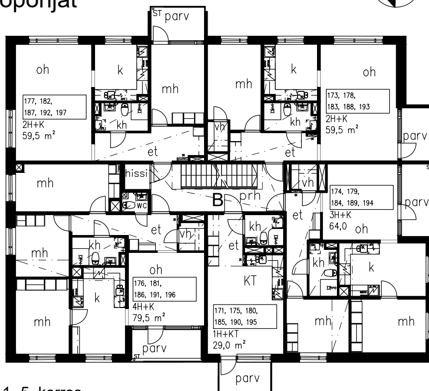
1.-5. kerros
